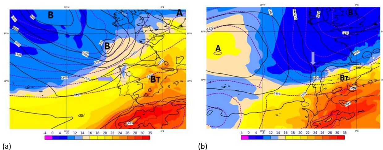
Figura 2 - Tipos de Tempo agosto de 2023: ECMWF(ERA5), pressão ao nível médio do mar (linhas a preto, hPa), altura do geopotencial aos 500 hPa (linhas violeta a tracejado, 50 em 50 m), temperatura aos 850 hPa (cor). (a) Tipo de tempo - W (Fluxo de oeste, 18 agosto), (b) Tipo de Tempo - N (Fluxo de norte, 26 agosto). A- Anticiclone, B- Depressão, BT- Depressão Térmica, seta a violeta - direção do fluxo.
