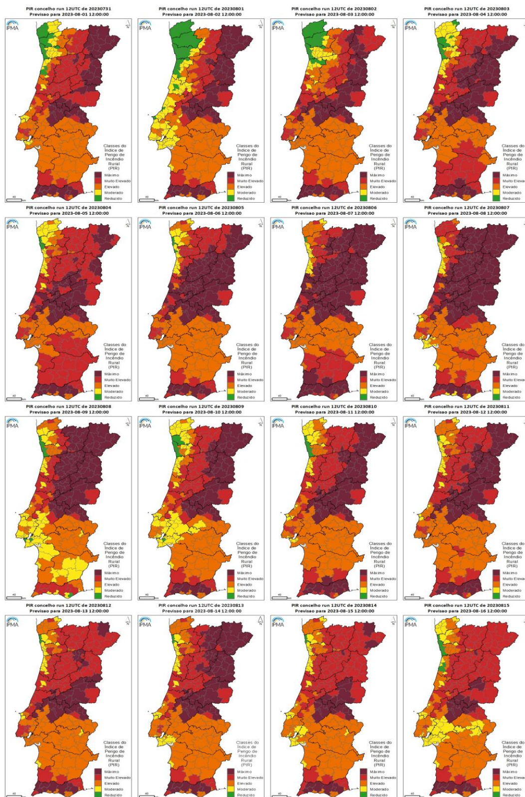
Figura AIII.3 – Mapas das classes de PIR, previsão a nível de Concelho, agosto de 2023 (dias 1 a 16).
