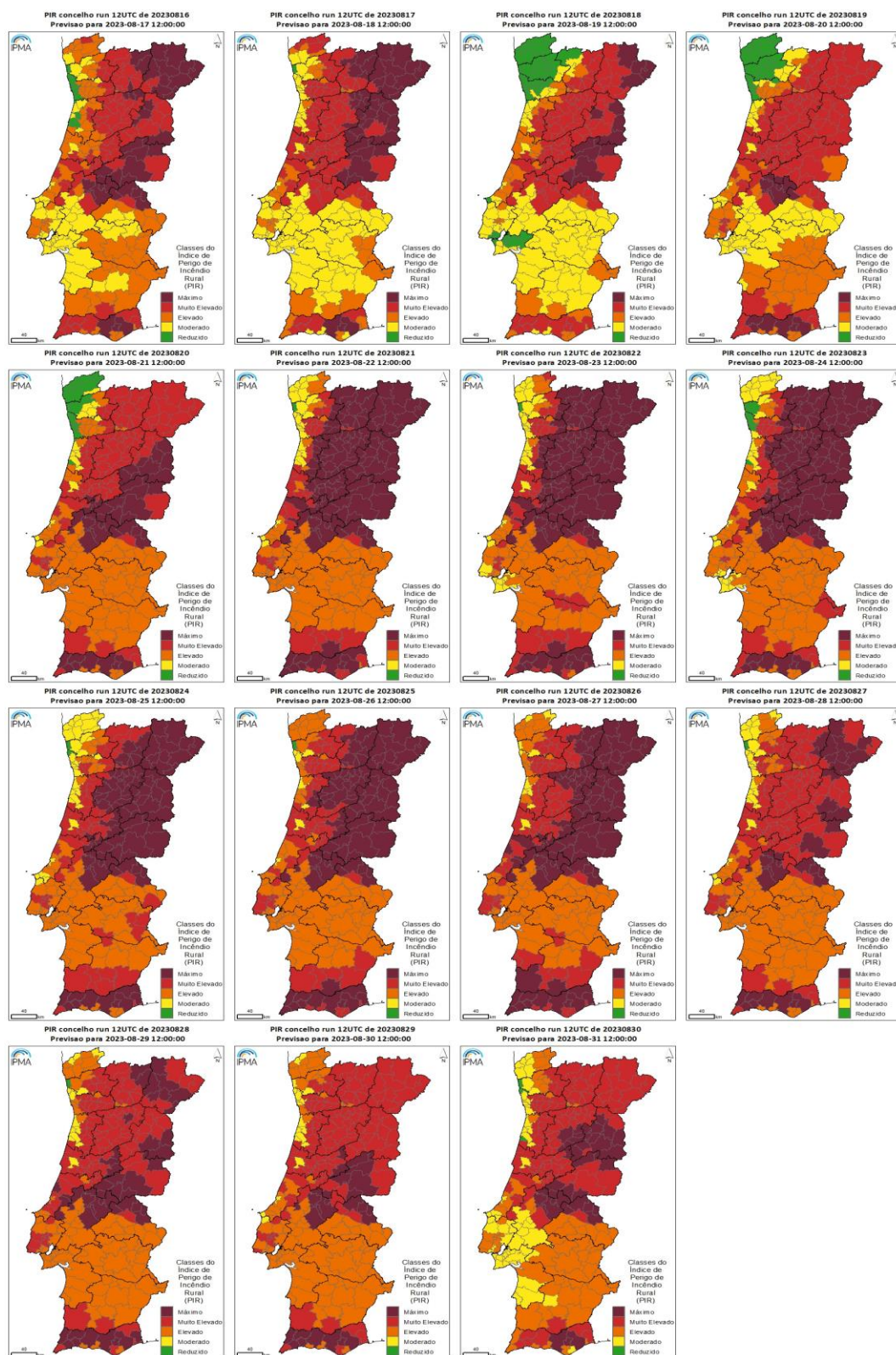
Figura AIII.4 – Mapas das classes de PIR, previsão a nível de Concelho, agosto de 2023 (17 a 31).
