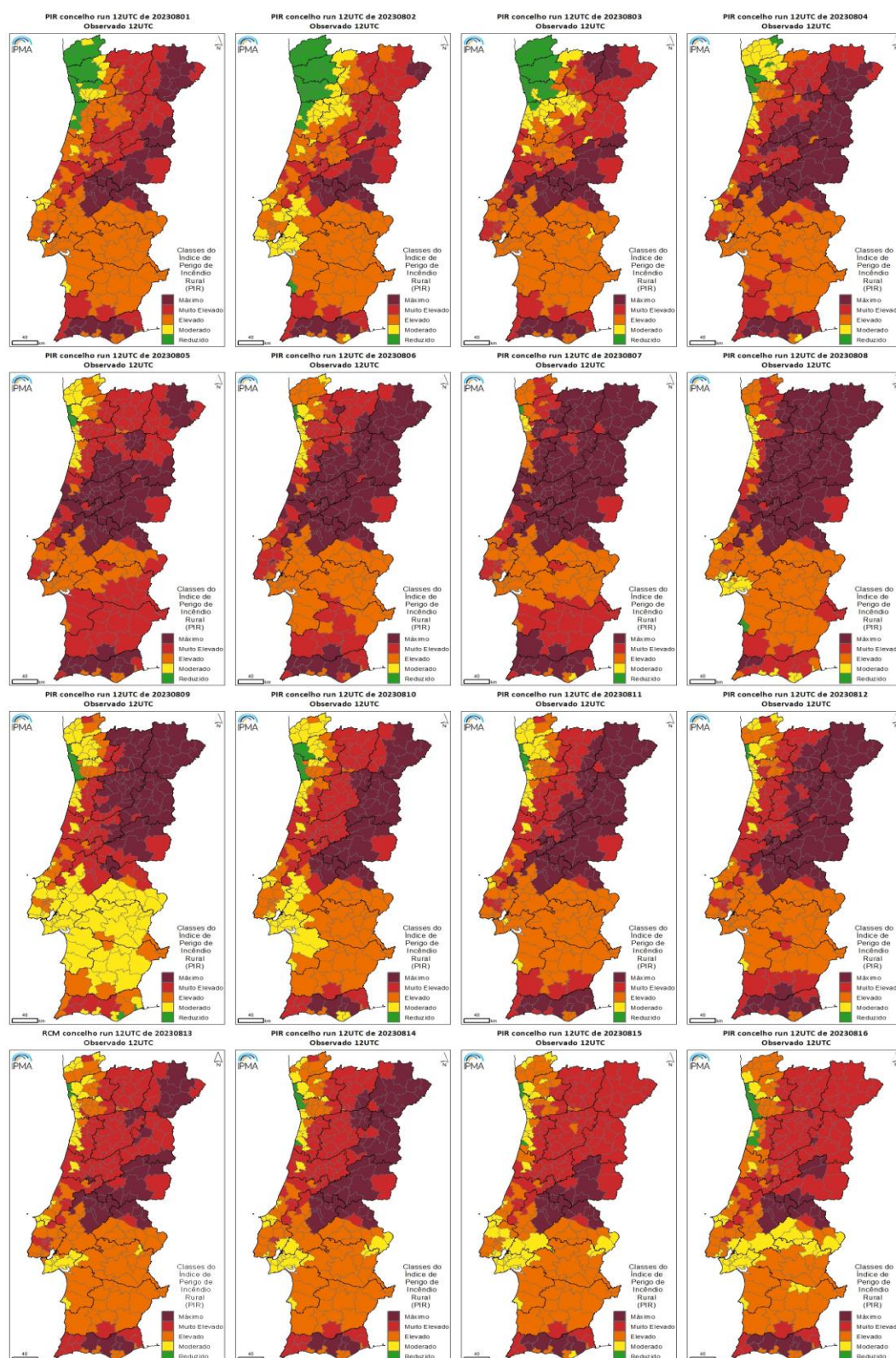
Figura AIII.1 – Mapas das classes do PIR observado a nível de Concelho, agosto de 2023 (dias 1 a 16).
