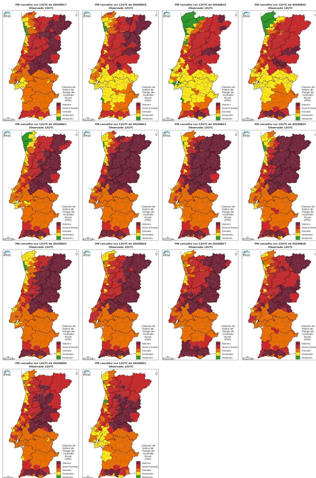
Figura AIII.2 – Mapas das classes de PIR observado a nível de Concelho, agosto de 2023 (dias 17 a 31).
