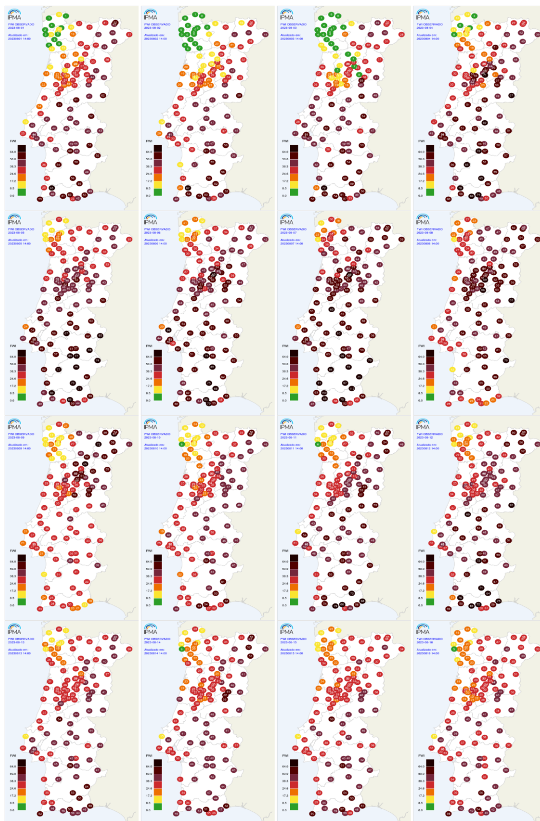
Figura AII.1 – Mapas do FWI Observado nas estações meteorológicas, agosto de 2023 (dias 1 a 16).
