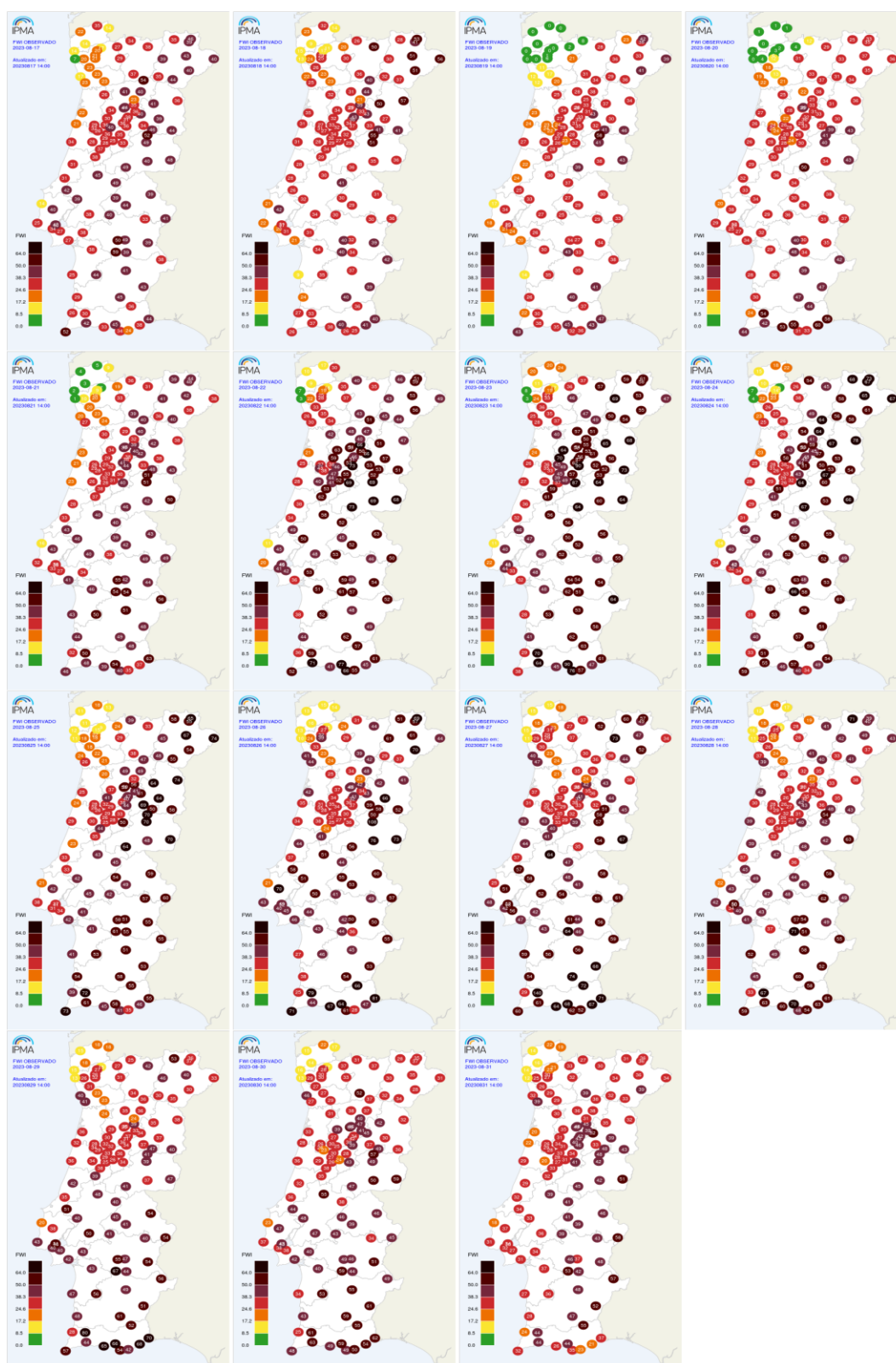
Figura AII.2 – Mapas do FWI Observado nas estações meteorológicas, agosto de 2023 (dias 17 a 31).
