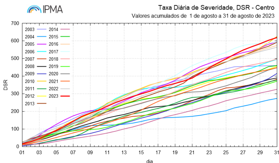
Figura 8 (b) – Evolução dos valores acumulados da taxa diária de severidade, DSR, no mês de agosto nos anos de 2003 a 2023.
