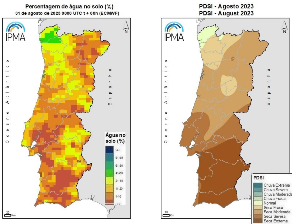
Figura 4 - Distribuição espacial em 31 de agosto de 2023 do teor de Água no Solo e da Seca, (a) percentagem de água no solo (média 0-100 cm profundidade), em relação à capacidade de água utilizável pelas plantas (ECMWF), (b) índice de seca, PDSI.
