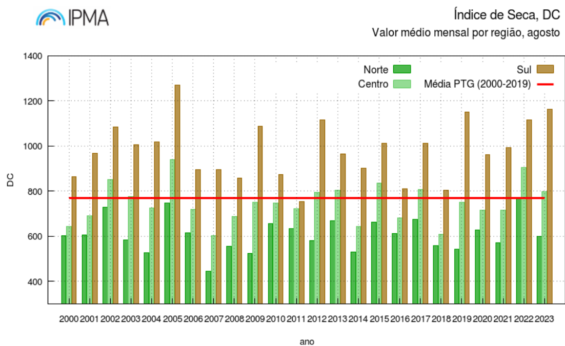
Figura 5 - Valor médio dos índices de seca, DC.
