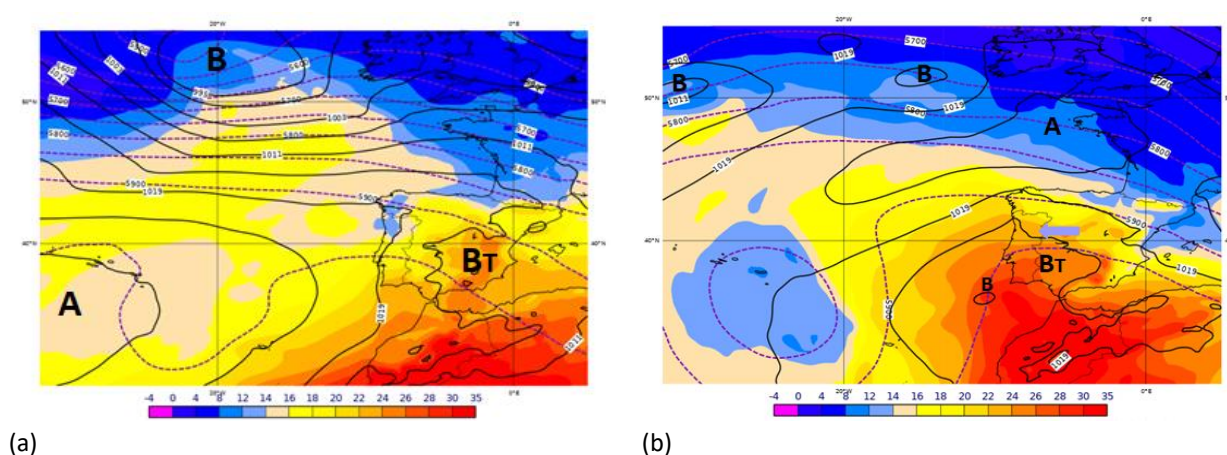
Figura 1 - Tipos de Tempo em agosto de 2023: ECMWF(ERA5), pressão ao nível médio do mar (linhas a preto, hPa), altura do geopotencial aos 500 hPa (linhas violeta a tracejado, 50 em 50 m), temperatura aos 850 hPa (cor). (a) Tipo de Tempo – A (Anticiclónico, 1 agosto), (b) Tipo de Tempo – E (fluxo de leste, 7 agosto). A- Anticiclone, B- Depressão, B T - Depressão Térmica, seta a violeta - direção do fluxo.
