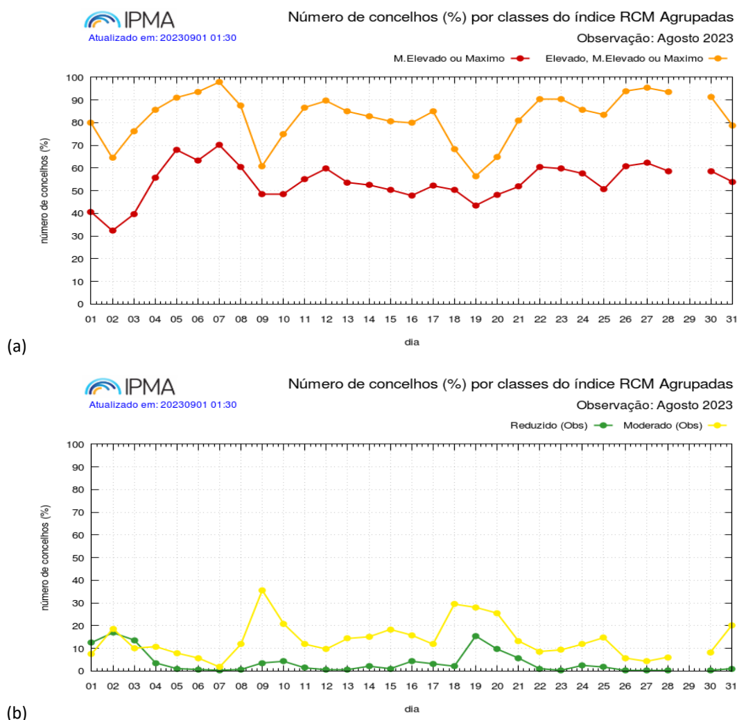
Figura 9 - Evolução diária em setembro da percentagem de concelhos nas classes de PIR. (a) Elevado Muito Elevado ou Máximo (laranja), Muito Elevado ou Máximo (vermelho), (b) Reduzido (verde), Moderado (amarelo).
