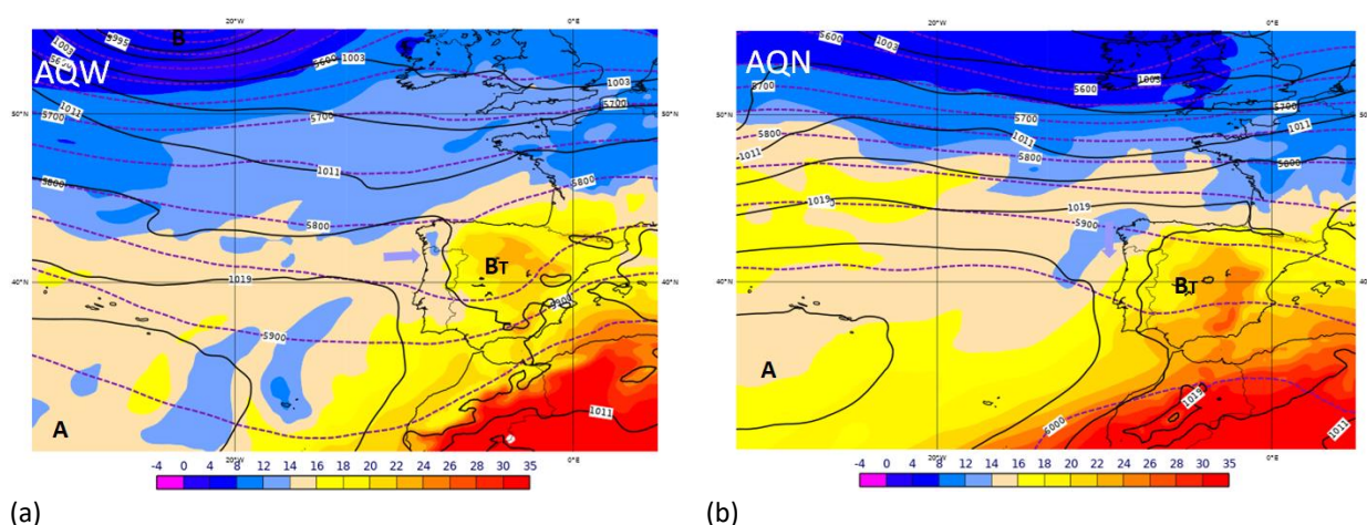
Figura 2 - Tipos de Tempo julho de 2023: ECMWF(ERA5), pressão ao nível médio do mar (linhas a preto, hPa), altura do geopotencial aos 500 hPa (linhas violeta a tracejado, 50 em 50 m), temperatura aos 850 hPa (cor). (a) Tipo de tempo - AQW (Anticiclónico e Fluxo quadrante oeste, 27julho), (b) Tipo de Tempo - AQN (Anticiclónico e Fluxo do quadrante norte, 31 julho). A- Anticiclone, B- Depressão, B T Depressão Térmica, seta a violeta - direção do fluxo.
