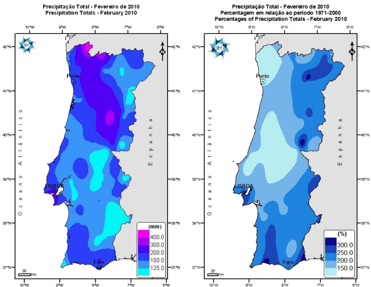
Figura 4 Precipitação total em Fevereiro (esq.) e respectiva percentagem em relação à média 1971-2000 (dir.).
