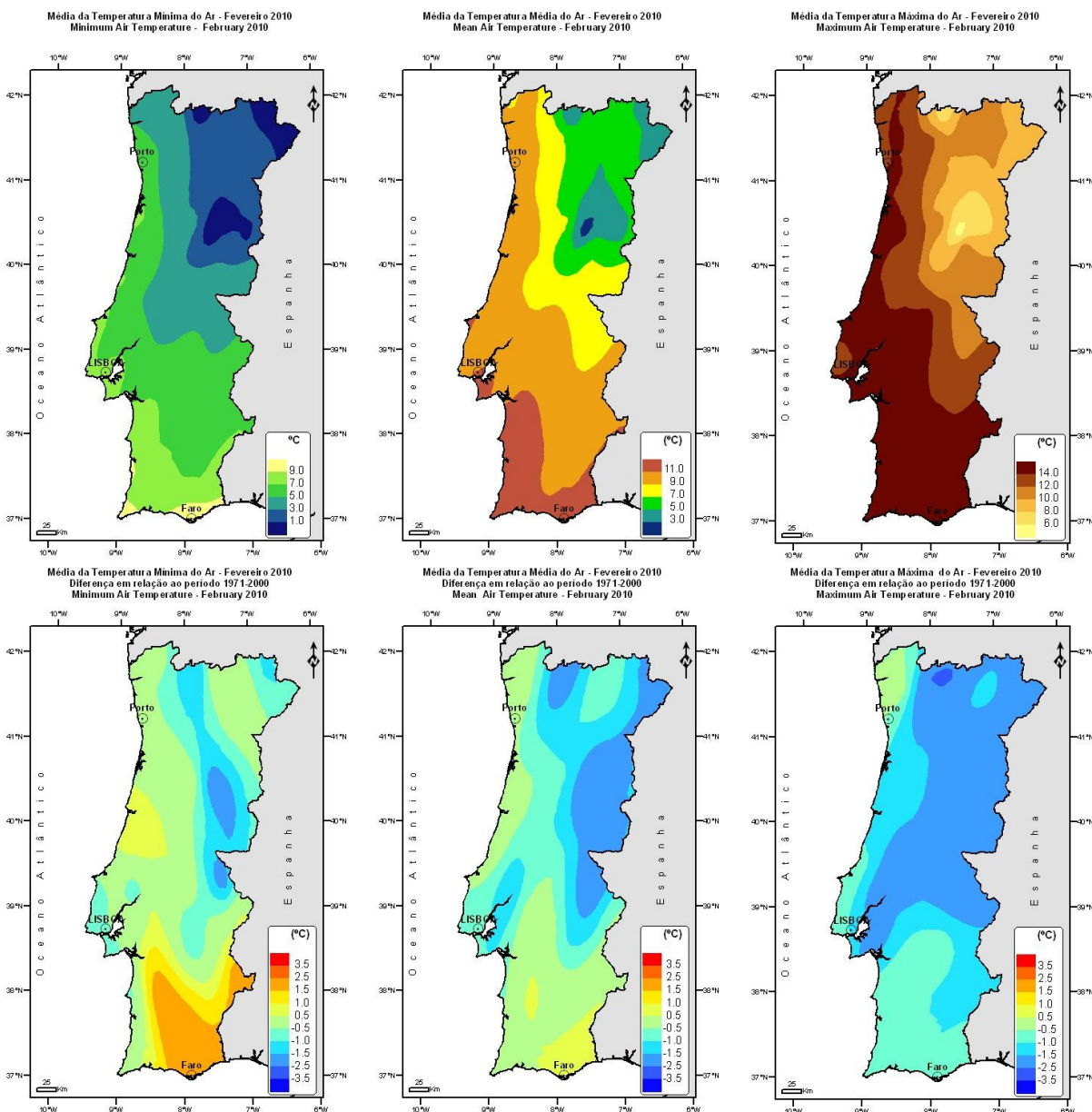
Figura 3 Distribuição espacial da temperatura mínima, média e máxima do ar em Fevereiro e respectivos desvios em relação à média 1971-2000
