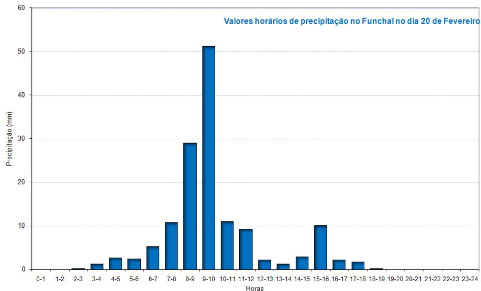
Figura 1- Valores acumulados de precipitação em 1 hora entre as 00 e as 24h do dia 20 de Fevereiro no Funchal
