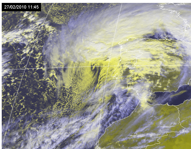
Figura 10 - Imagem combinada de alta resolução do satélite MSG às 11:45 UTC de dia 27/02/2010
