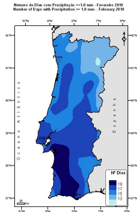
Figura 11 - Número de dias com precipitação superior ou igual a 1mm em Fevereiro de 2010
