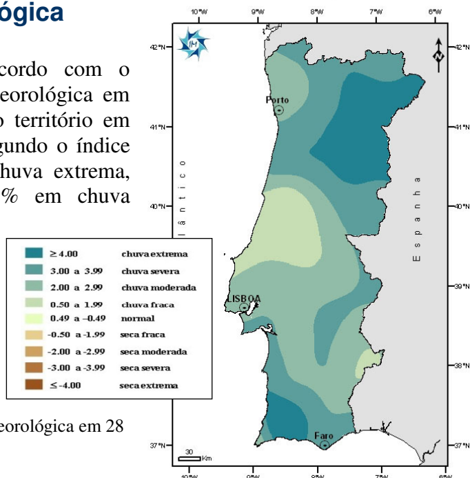
PDSI - Fevereiro de 2010 PDSI - February 2010
