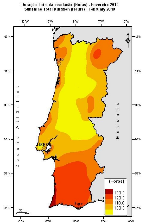
Figura 6 Insolação em Fevereiro 2010
