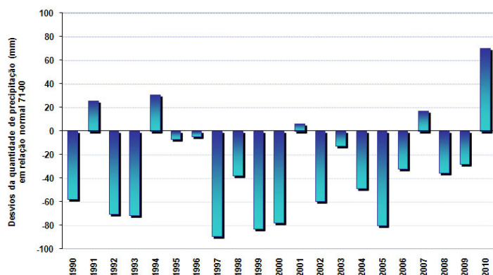
Figura 2 Precipitação Total em Fevereiro (esq.2a) e temperatura máxima em Fevereiro em Portugal Continental (dir.2b). Desvios em relação à média 1971-2000
