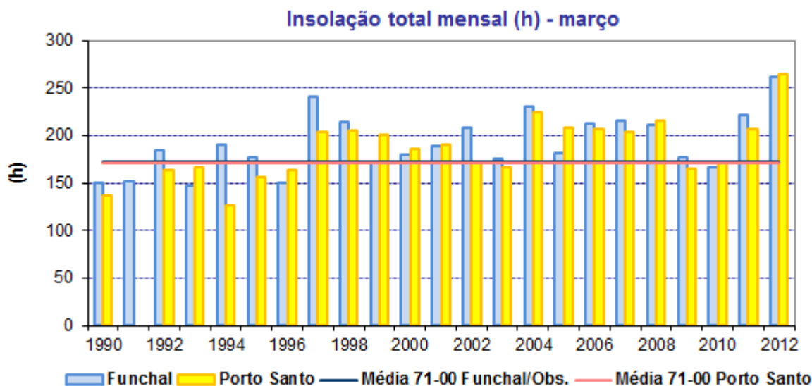
Figura 6. Insolação para os meses de março na estação do Funchal/Observatório e Porto Santo/Aeroporto (1990-2012) e valores médios 1971-2000.
