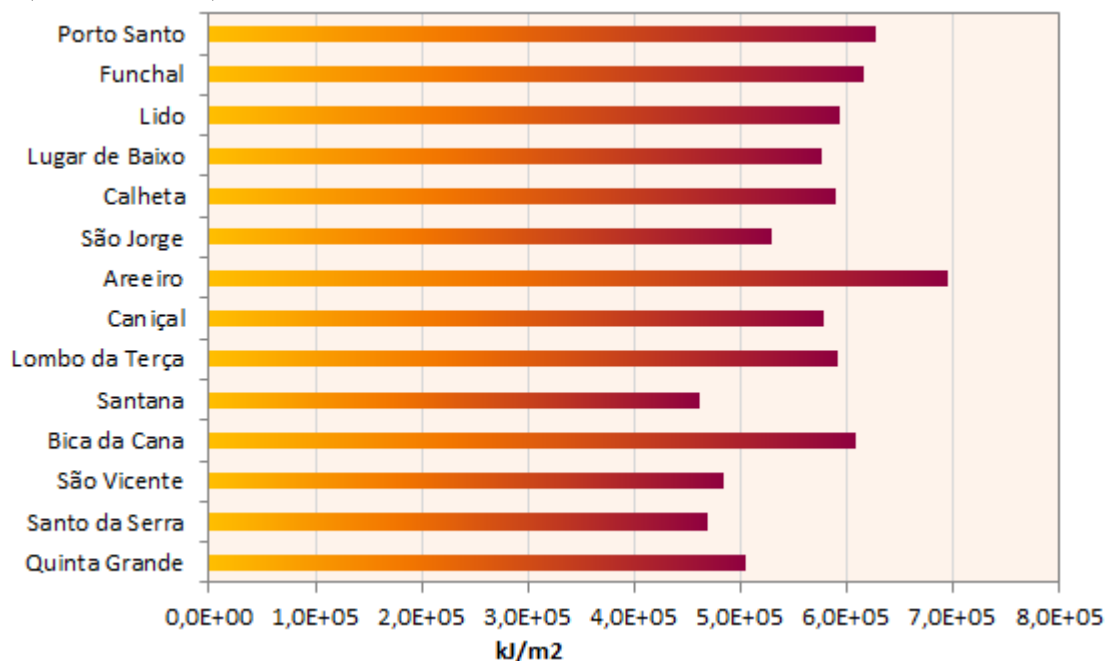
Figura 5. Radiação solar global mensal nas estações do Arquipélago da Madeira para o mês de março.
