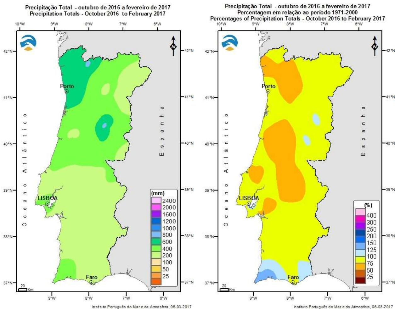
Figura 7 - Precipitação acumulada desde 1 de outubro 2016 (esq.) e percentagem em relação à média 1971-2000 (dir.)
