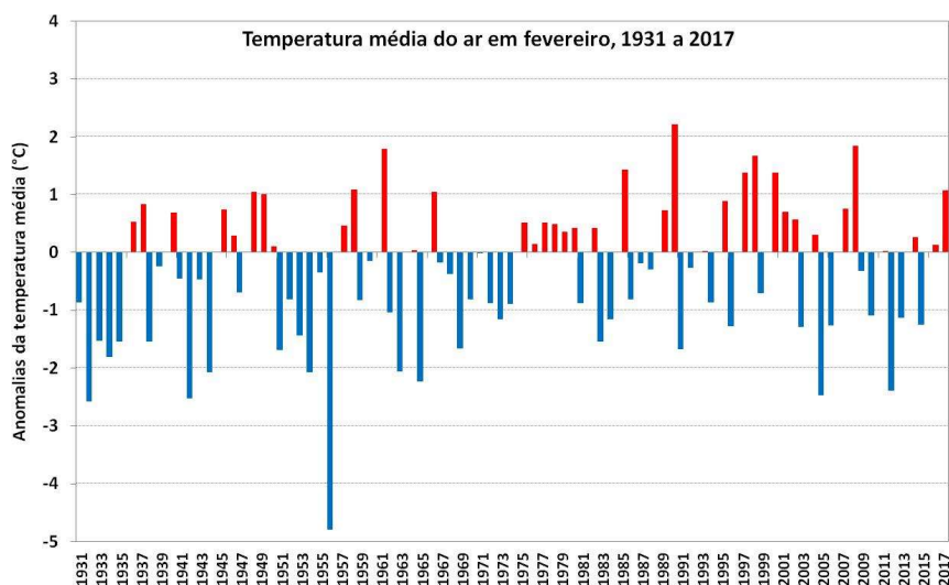
Figura 2- Anomalias da temperatura média do ar em relação aos valores médios no período 1971-2000, no mês de fevereiro, em Portugal continental.
