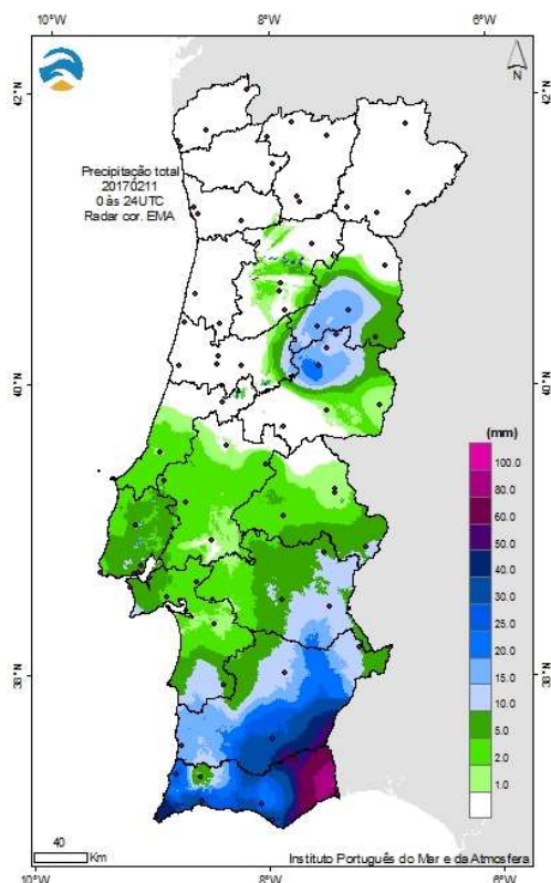
Figura 9 - Precipitação acumulada (mm) em 24 horas, no dia 11 de fevereiro 2017 estimada através do método combinado de ajustamento radar/udómetro
