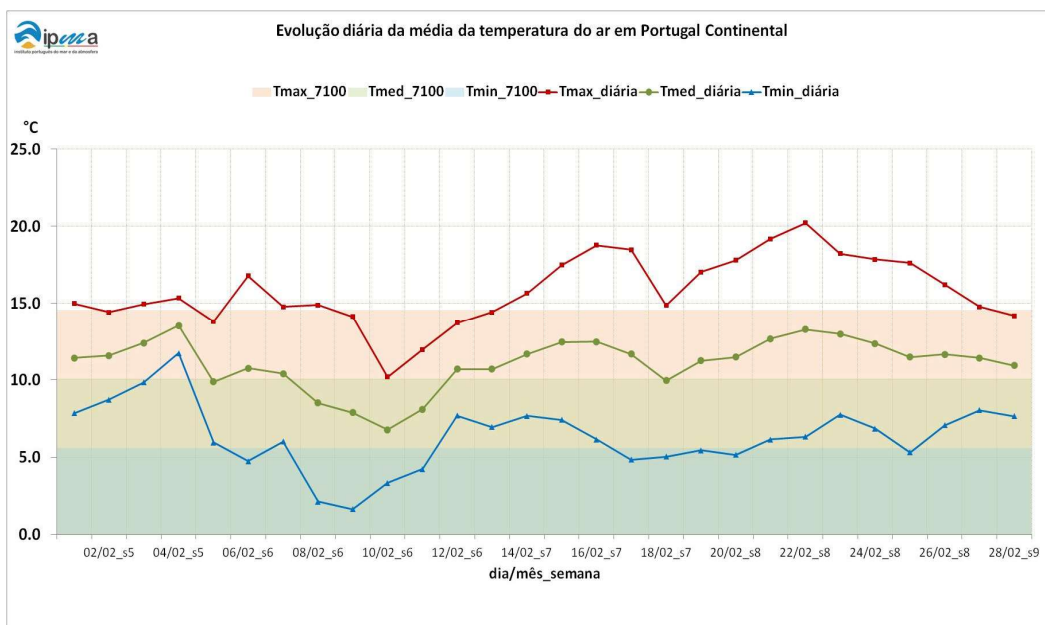
Figura 1 – Evolução diária da temperatura do ar de 1 a 28 de fevereiro de 2017 em Portugal Continental. (Tmax, Tmed e Tmin designam, respetivamente, temperatura máxima, média e mínima).
