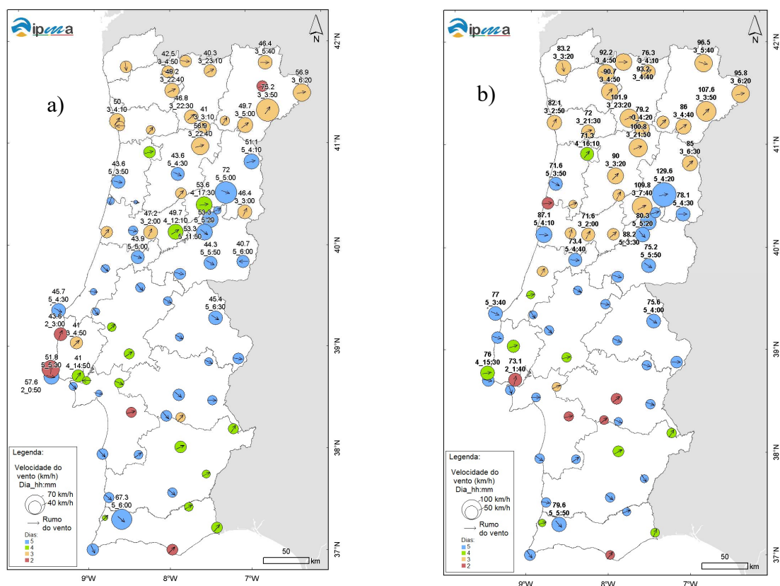
Figura 8 – Valores máximos de velocidade instantânea do vento (a) e de vento médio (b) e respetivo rumo, na rede de observação do IPMA no período de 2 a 5 de fevereiro de 2017
