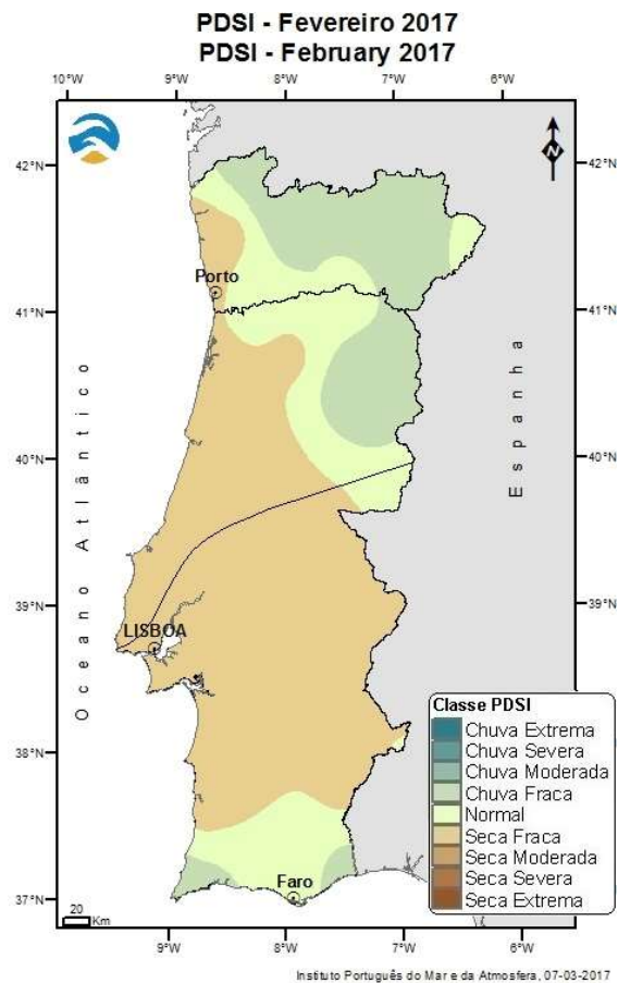
Figura 10 – Distribuição espacial do índice de seca meteorológica a 28 de fevereiro de 2017
