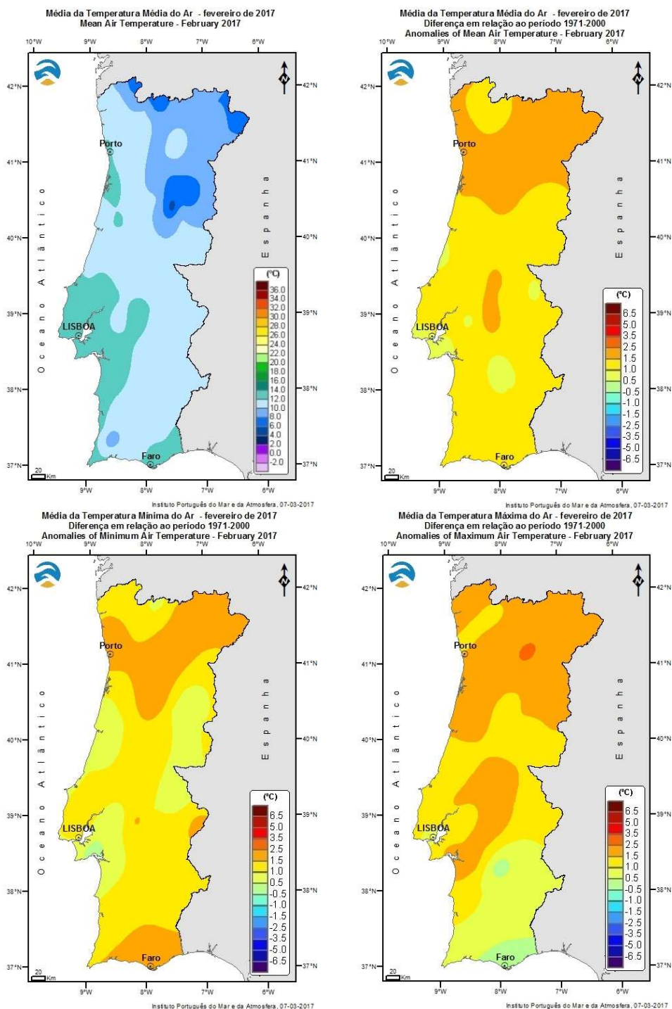
Figura 4 - Distribuição espacial dos valores médios da temperatura média do ar e anomalias da temperatura média, mínima e máxima do ar (em relação ao período 1971-2000), no mês de fevereiro.
