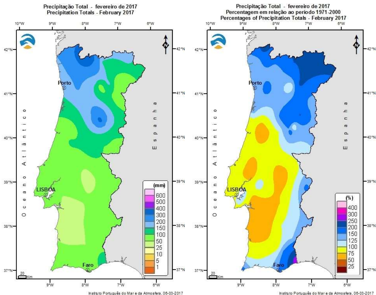
Figura 6 – Distribuição espacial da precipitação total e respetiva percentagem em relação à média em fevereiro.
