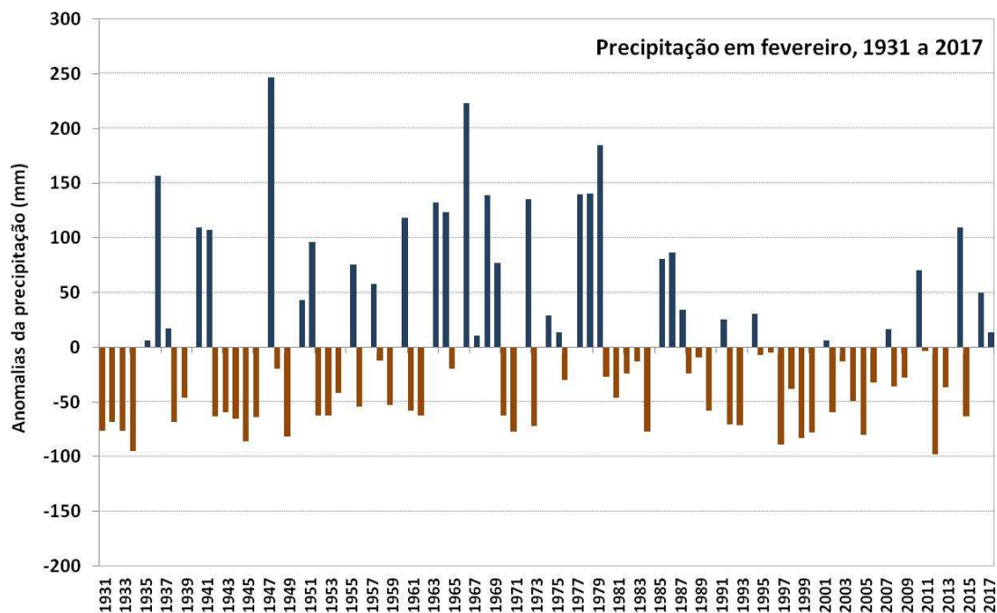
Figura 5- Anomalias da quantidade de precipitação em relação aos valores médios no período 1971-2000, no mês de fevereiro, em Portugal continental.
