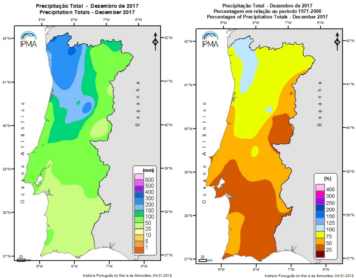
Figura 6 – Distribuição espacial da precipitação total e respetiva percentagem em relação à média em dezembro.
