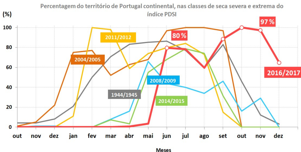
Figura 9 – Evolução mensal da percentagem do território em seca severa e extrema, de acordo com a classificação do índice PDSI, para várias situações de seca (histórica:1944/45; após 2000: 2004/05, 2008/09, 2011/12, 2014/15 e 2016/17)
