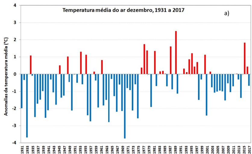
Figura 1 - Anomalias da temperatura média (a) e anomalias da quantidade de precipitação (b) em dezembro, em Portugal continental, em relação aos valores médios no período 1971-2000
