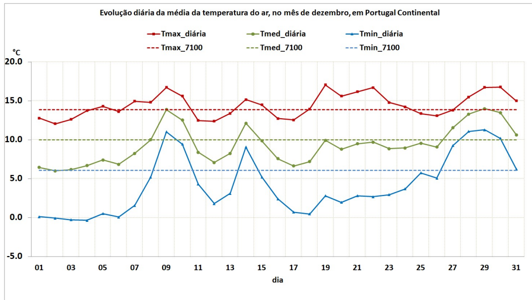
Figura 4 – Evolução diária da temperatura do ar de 1 a 31 de dezembro de 2017 em Portugal continental. (Tmax, Tmed e Tmin designam, respetivamente, temperatura máxima, média e mínima).
