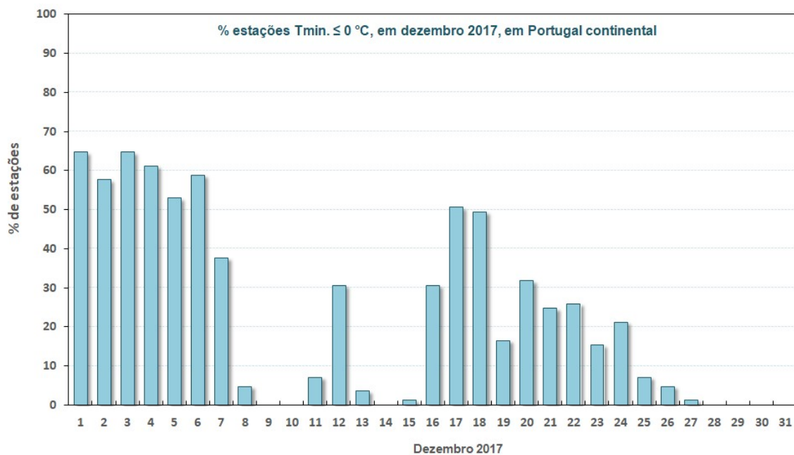
Figura 5 – Percentagem de estações com valores de mínima \leq 0\text{ }^{\circ}\text{C} , em dezembro 2017 em Portugal continental (total de estações: 85)
