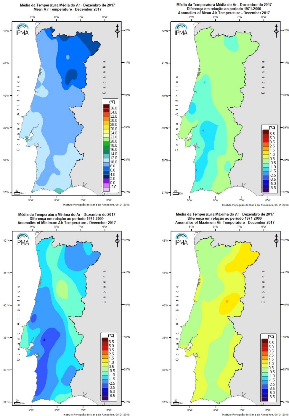
Figura 3 - Distribuição espacial dos valores médios da temperatura média do ar e anomalias da temperatura média, mínima e máxima do ar (em relação ao período 1971-2000), no mês de dezembro.
