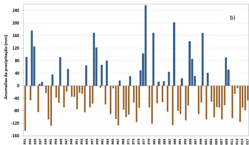
Figura 1 - Anomalias da temperatura média (a) e anomalias da quantidade de precipitação (b) em dezembro, em Portugal continental, em relação aos valores médios no período 1971-2000
