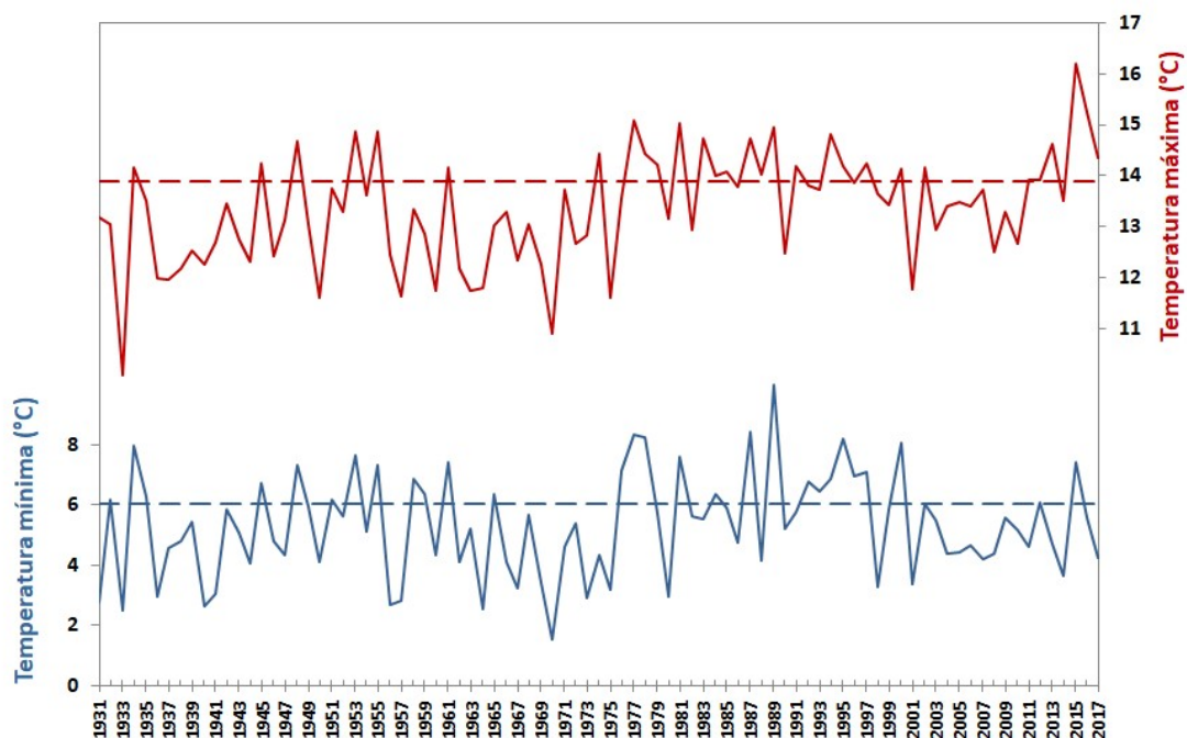
Figura 2 – Variabilidade da temperatura máxima e mínima do ar em dezembro, em Portugal continental. (Linhas a tracejado indicam a média no período 1971-2000)
