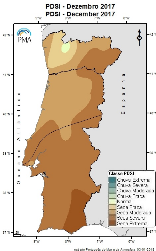
Figura 8 – Distribuição espacial do índice de seca meteorológica a 31 de dezembro de 2017
