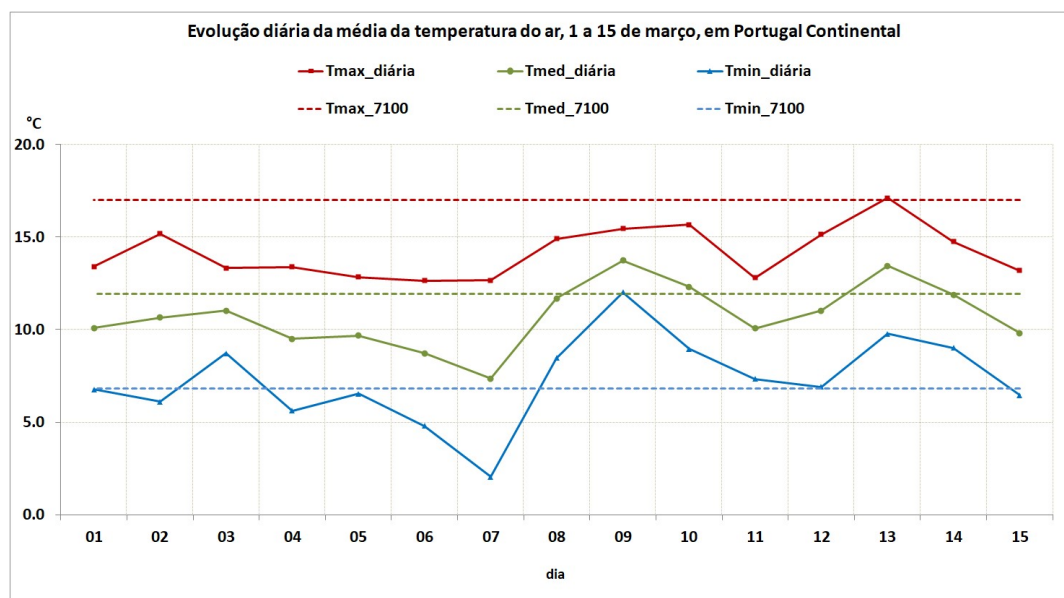
Figura 6 – Evolução diária da temperatura (máxima, média e mínima do ar) do ar de 1 a 15 de março de 2018 em Portugal continental e respetivos valores médios 1971-2000
