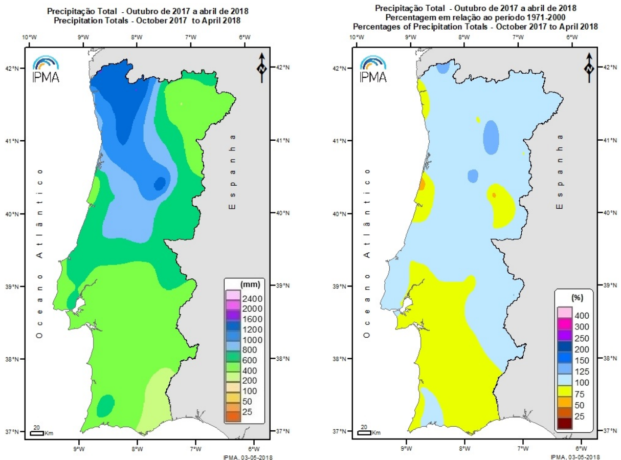
Figura 6 - Precipitação acumulada desde 1 de outubro 2017 (esq.) e percentagem em relação à média 1971-2000 (dir.)
