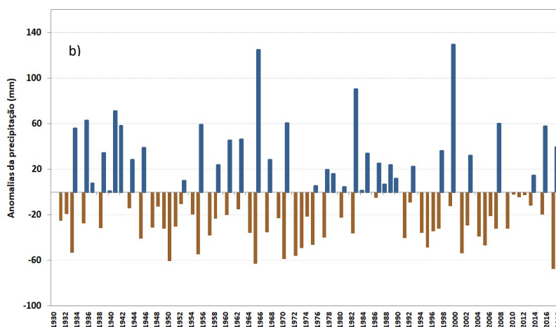
Figura 1 - Anomalias da temperatura média (a) e anomalias da quantidade de precipitação (b) em abril, em Portugal continental, em relação aos valores médios no período 1971-2000
