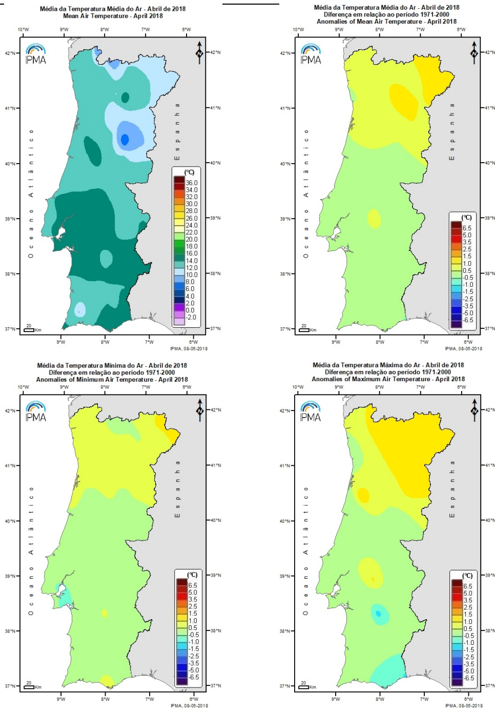
Figura 3 - Distribuição espacial dos valores médios da temperatura média do ar e anomalias da temperatura média, mínima e máxima do ar (em relação ao período 1971-2000), no mês de abril de 2018.
