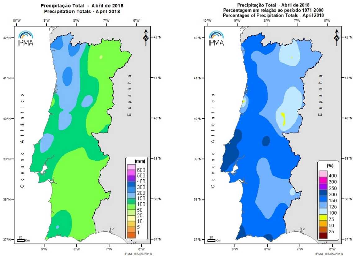
Figura 5 – Distribuição espacial da precipitação total e respetiva percentagem em relação à média em abril
