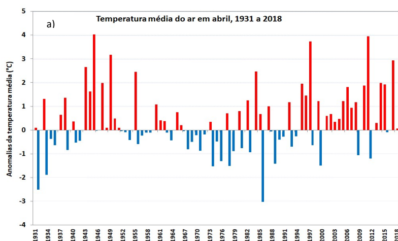
Figura 1 - Anomalias da temperatura média (a) e anomalias da quantidade de precipitação (b) em abril, em Portugal continental, em relação aos valores médios no período 1971-2000
