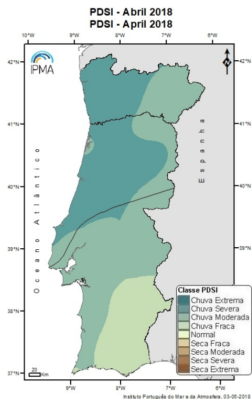
Figura 7 – Distribuição espacial do índice de seca meteorológica a 30 de abril de 2018
