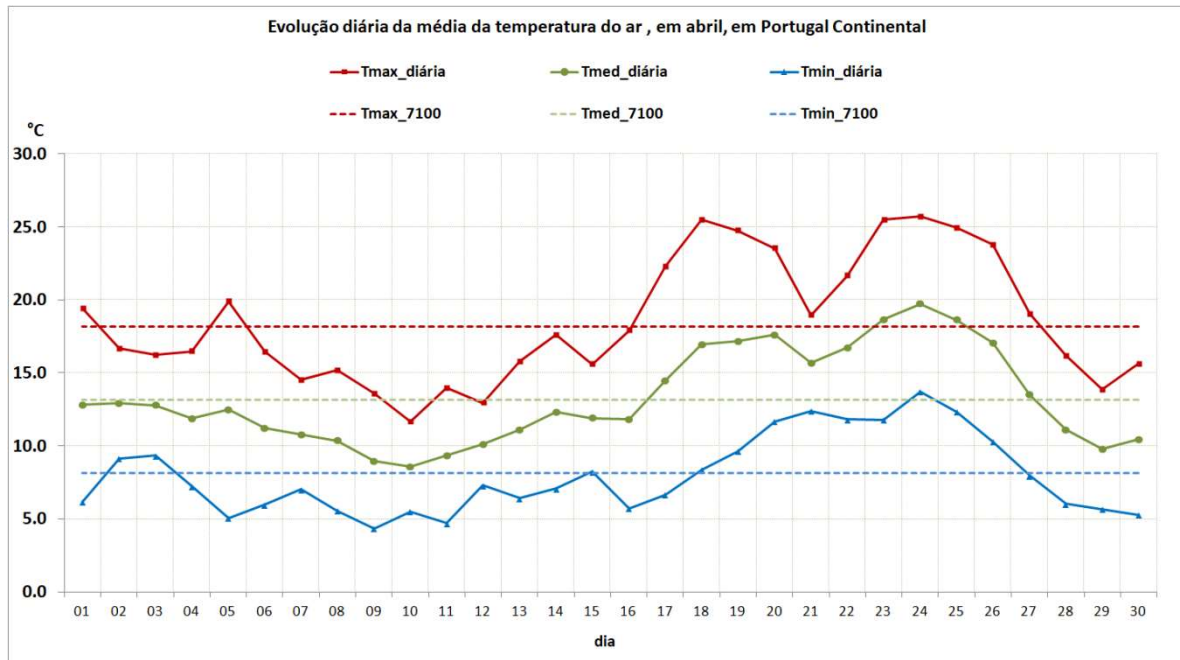
Figura 4 – Evolução diária da temperatura (máxima, média e mínima do ar) do ar de 1 a 30 de abril de 2018 em Portugal continental e respetivos valores médios 1971-2000
