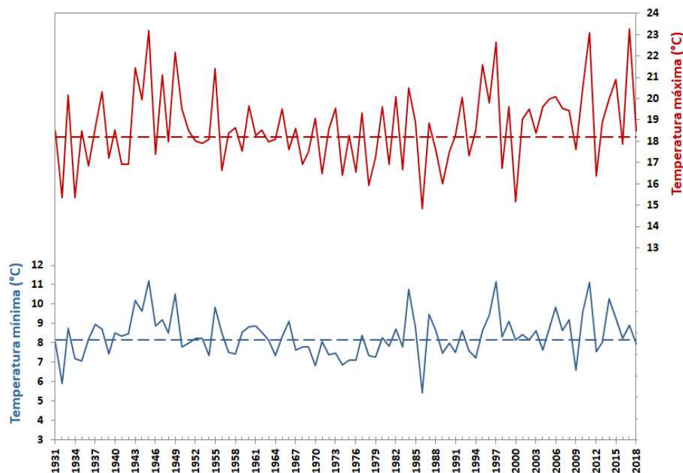
Figura 2 – Variabilidade da temperatura máxima e mínima do ar no mês de abril, em Portugal continental. (Linhas a tracejado indicam a média no período 1971-2000)
