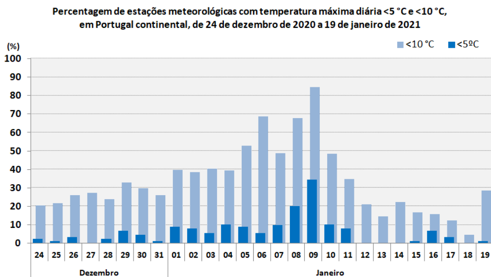
Figura 10 - Evolução diária da percentagem de estações meteorológicas com temperatura máxima do ar inferior a 5 °C e 10 °C em Portugal continental, de 24 de dezembro de 2020 a 19 de janeiro de 2021.
