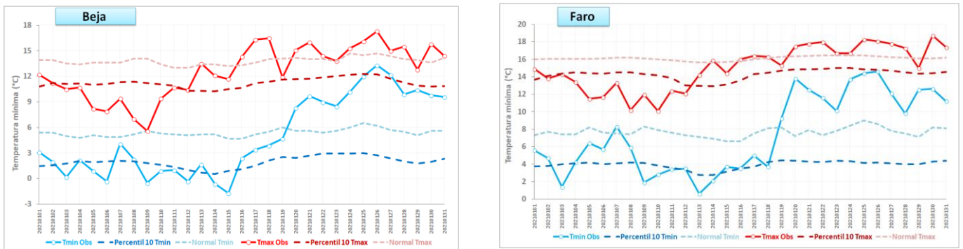
Figura 11 - Valores diários da temperatura mínima e máxima, respetivo percentil 10 e valor médio diário em janeiro 2021
