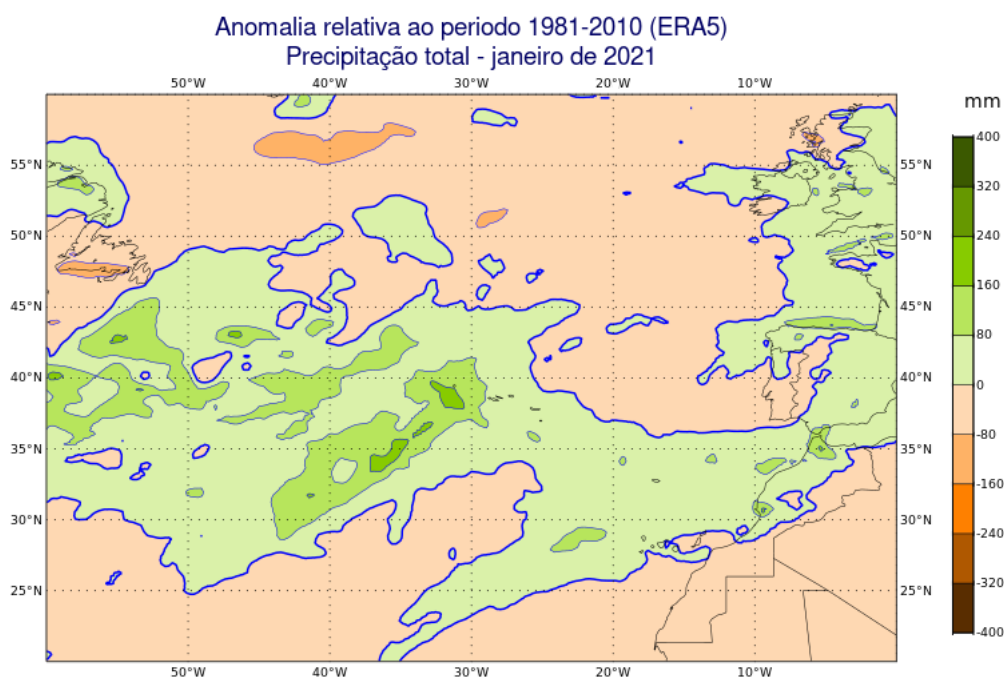
Figura 13 – Anomalia da precipitação total em janeiro 2021
