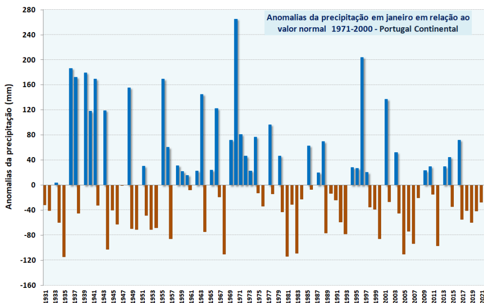
Figura 14 – Anomalias da quantidade de precipitação, no mês de janeiro, em Portugal continental, em relação aos valores médios no período 1971-2000
