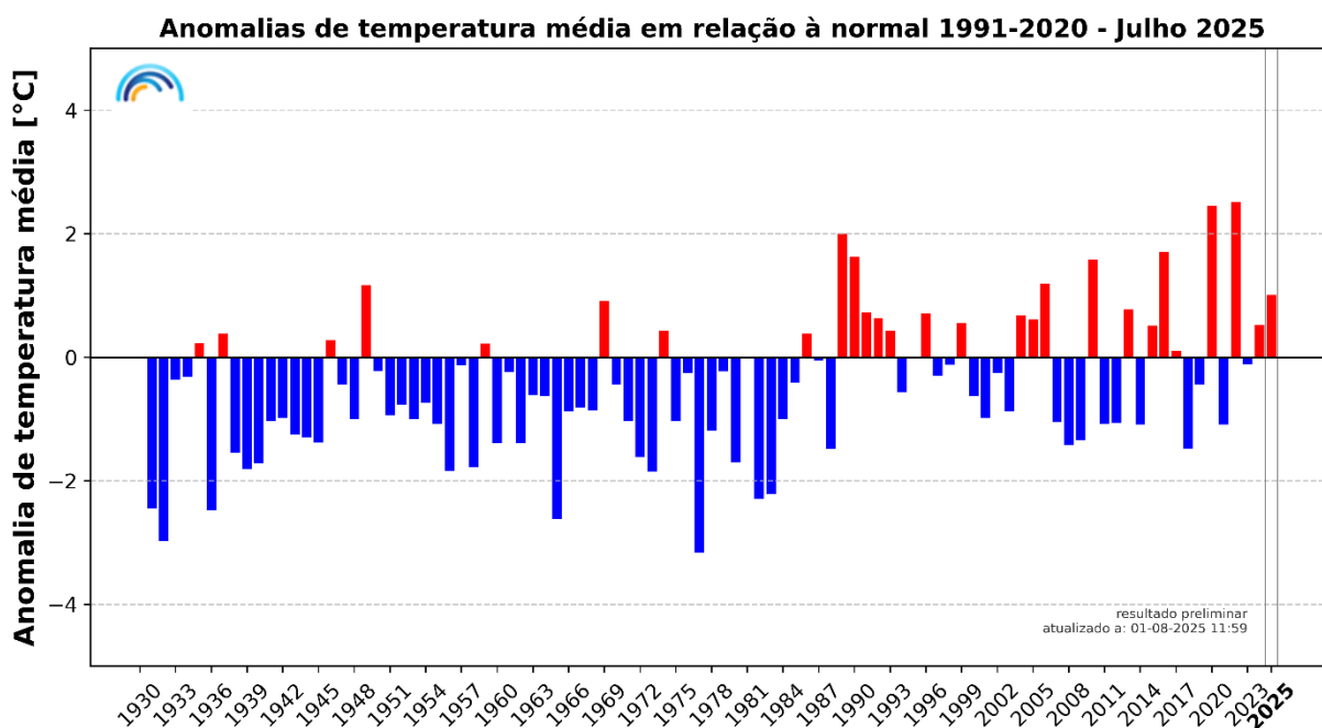
Figura 2. Anomalias da temperatura média do ar de julho 2025, em Portugal continental, em relação aos valores médios 1991-2020. Foram utilizadas, nesta análise preliminar, 98% das estações meteorológicas da rede do IPMA.
