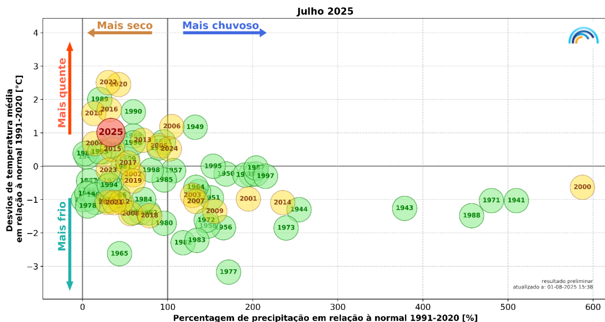
Figura 1. Desvio da temperatura média do ar e percentagem da precipitação (em relação à normal 91-20) de julho em Portugal continental entre 1941 e 2025.
