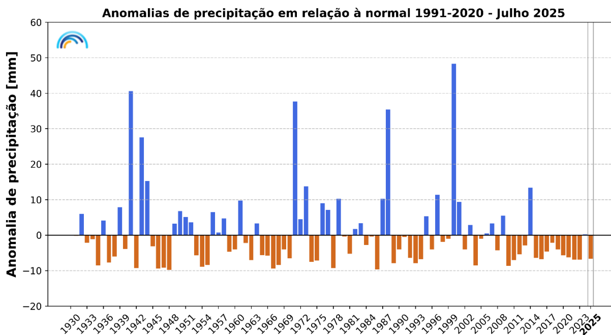
Figura 3. Anomalias da quantidade de precipitação de julho 2025 em Portugal continental, em relação ao valor médio 1991-2020. Foram utilizadas, nesta análise preliminar, 95 % das estações meteorológicas da rede do IPMA.
