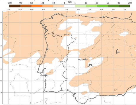
ECMWF - Anomalia Semanal da precipitação total Previsão de 20250528, válida para semana de 20250616 00H00 a 20250623 00h00
