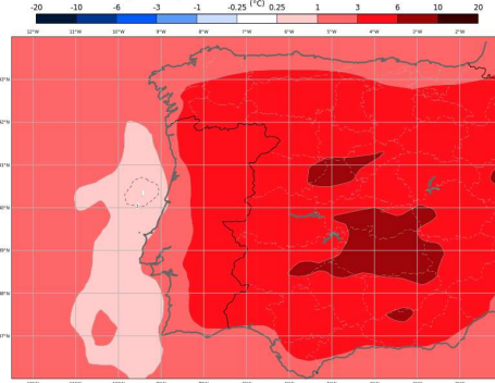
ECMWF - Anomalia Semanal da Temperatura a 2 metros Previsão de 20250528, válida para semana de 20250609 00H00 a 20250616 00h00
