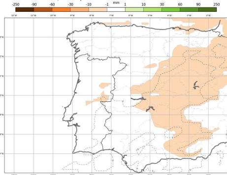
ECMWF - Anomalia Semanal da precipitação total Previsão de 20250528, válida para semana de 20250623 00H00 a 20250630 00h00
