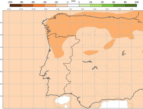
ECMWF - Anomalia Semanal da precipitação total Previsão de 20250528, válida para semana de 20250609 00H00 a 20250616 00h00
