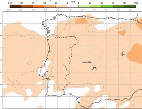
ECMWF - Anomalia Semanal da precipitação total Previsão de 20250528, válida para semana de 20250602 00H00 a 20250609 00h00
