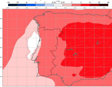
ECMWF - Anomalia Semanal da Temperatura a 2 metros Previsão de 20250528, válida para semana de 20250602 00H00 a 20250609 00h00
