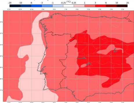
ECMWF - Anomalia Semanal da Temperatura a 2 metros Previsão de 20250528, válida para semana de 20250616 00H00 a 20250623 00h00
