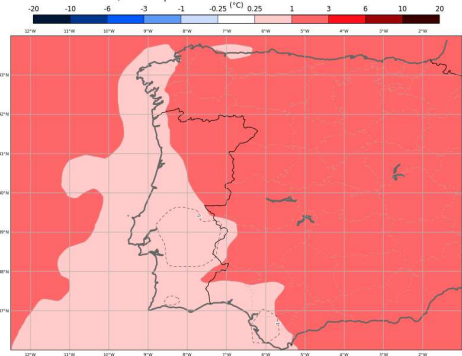
ECMWF - Anomalia Semanal da Temperatura a 2 metros Previsão de 20250528, válida para semana de 20250623 00H00 a 20250630 00h00
