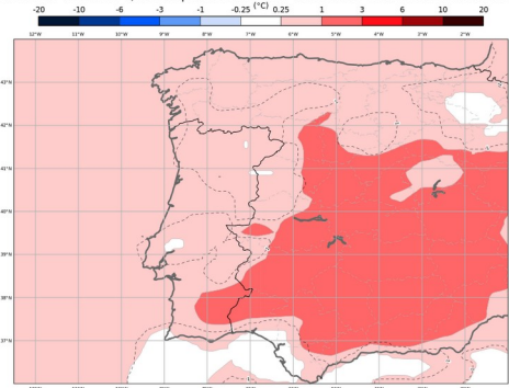
ECMWF - Anomalia Semanal da Temperatura a 2 metros Previsão de 20250514, válida para semana de 20250609 00H00 a 20250616 00h00
