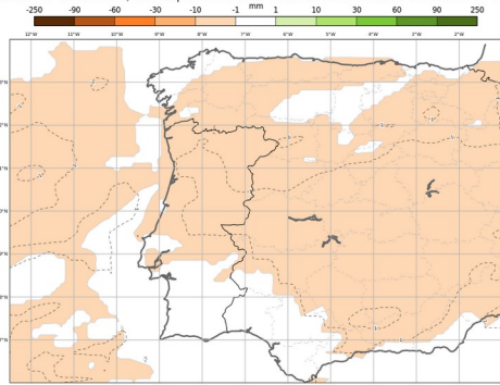
ECMWF - Anomalia Semanal da precipitação total Previsão de 20250514, válida para semana de 20250609 00H00 a 20250616 00h00
