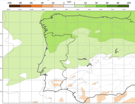
ECMWF - Anomalia Semanal da precipitação total Previsão de 20250514, válida para semana de 20250519 00H00 a 20250526 00h00
