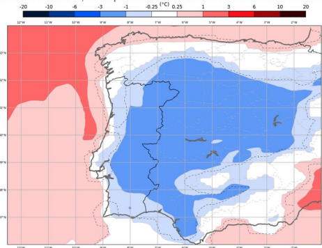
ECMWF - Anomalia Semanal da Temperatura a 2 metros Previsão de 20250514, válida para semana de 20250519 00H00 a 20250526 00h00
