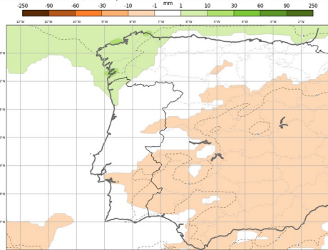
ECMWF - Anomalia Semanal da precipitação total Previsão de 20250514, válida para semana de 20250602 00H00 a 20250609 00h00
