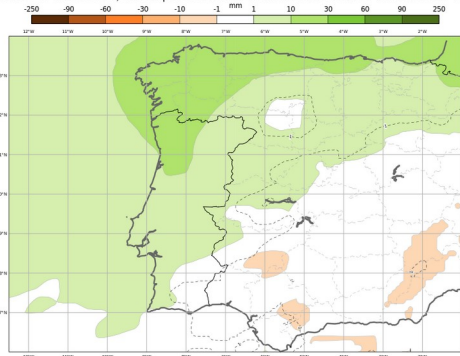
ECMWF - Anomalia Semanal da precipitação total Previsão de 20250514, válida para semana de 20250526 00H00 a 20250602 00h00
