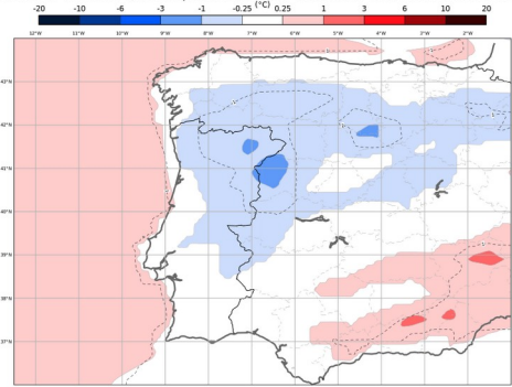
ECMWF - Anomalia Semanal da Temperatura a 2 metros Previsão de 20250514, válida para semana de 20250602 00H00 a 20250609 00h00
