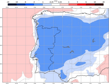
ECMWF - Anomalia Semanal da Temperatura a 2 metros Previsão de 20250514, válida para semana de 20250526 00H00 a 20250602 00h00
