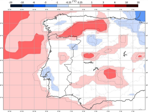
ECMWF - Anomalia Semanal da Temperatura a 2 metros Previsão de 20250108, válida para semana de 20250113 00H00 a 20250120 00h00
