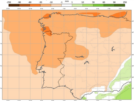
ECMWF - Anomalia Semanal da precipitação total Previsão de 20250108, válida para semana de 20250113 00H00 a 20250120 00h00
