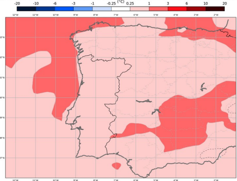
ECMWF - Anomalia Semanal da Temperatura a 2 metros Previsão de 20250108, válida para semana de 20250203 00H00 a 20250210 00h00
