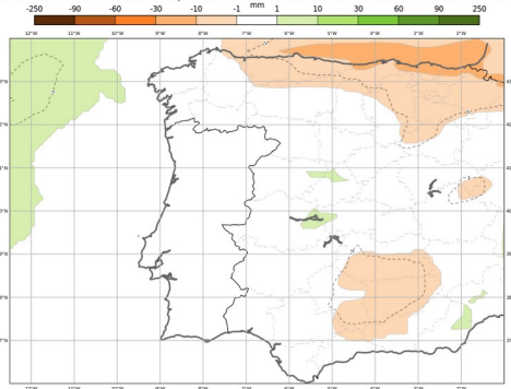
ECMWF - Anomalia Semanal da precipitação total Previsão de 20250108, válida para semana de 20250120 00H00 a 20250127 00h00
