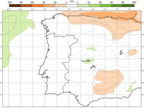
ECMWF - Anomalia Semanal da precipitação total Previsão de 20250108, válida para semana de 20250120 00H00 a 20250127 00h00
