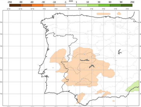
ECMWF - Anomalia Semanal da precipitação total Previsão de 20250108, válida para semana de 20250127 00H00 a 20250203 00h00
