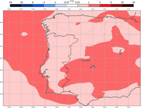
ECMWF - Anomalia Semanal da Temperatura a 2 metros Previsão de 20250108, válida para semana de 20250127 00H00 a 20250203 00h00
