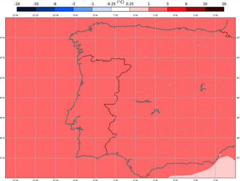
ECMWF - Anomalia Semanal da Temperatura a 2 metros Previsão de 20250108, válida para semana de 20250120 00H00 a 20250127 00h00
