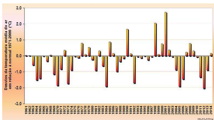
Temperatura média do ar
