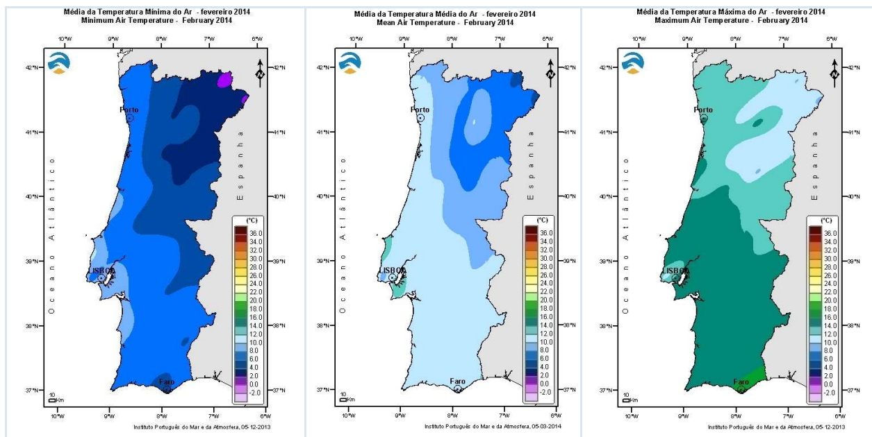
Figura 2 - Distribuição espacial dos valores médios da temperatura mínima, média e máxima do ar.
