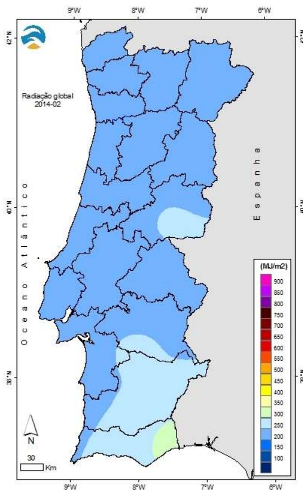
Figura 7 – Distribuição espacial dos valores da radiação solar global mensal ( \text{MJ}/\text{m}^2 ) em fevereiro de 2014
