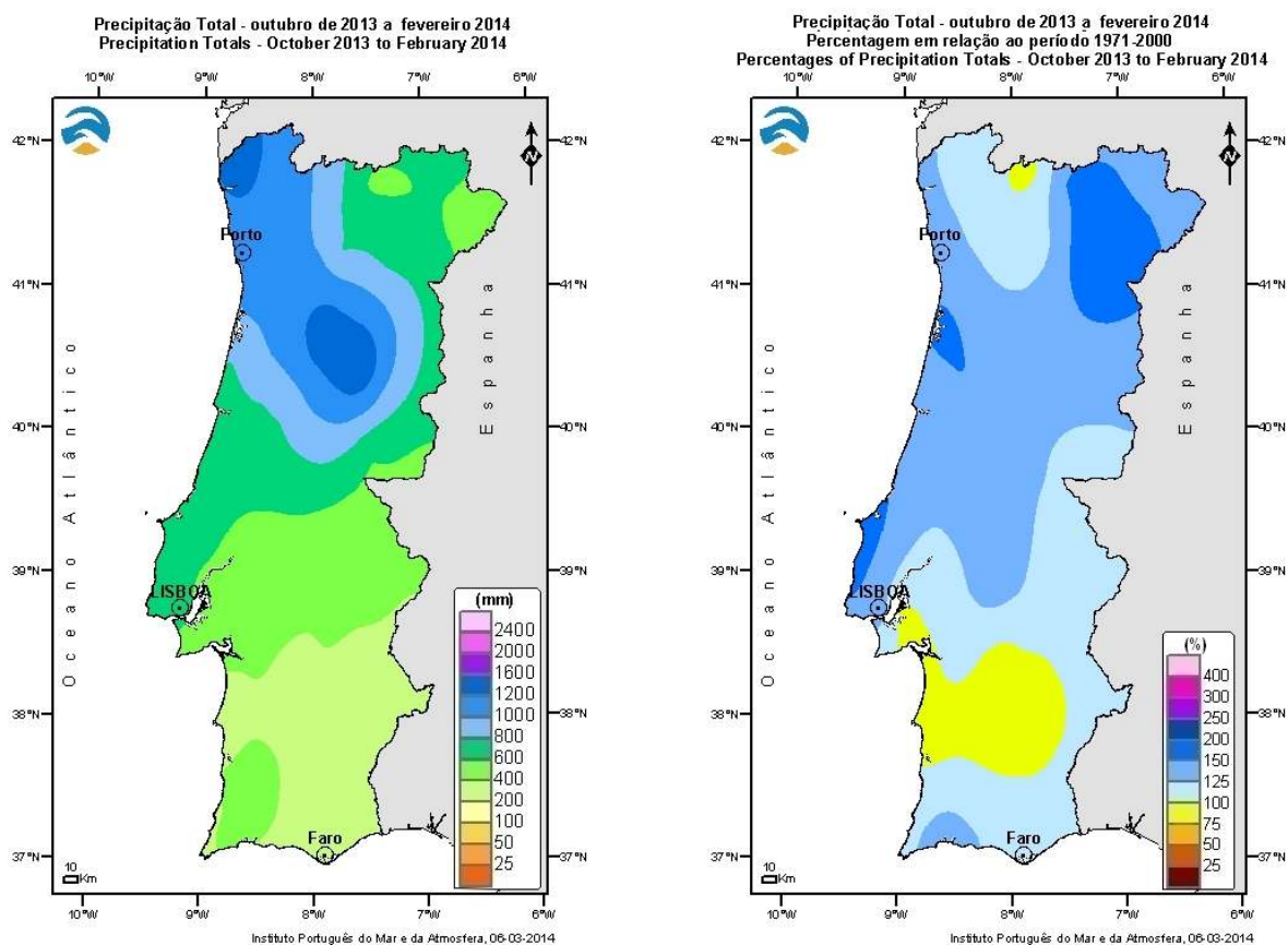
Figura 4 - Precipitação acumulada 1out – 28 fev 2014 (esq.) e percentagem em relação à média 1971-2000 (dir.)
