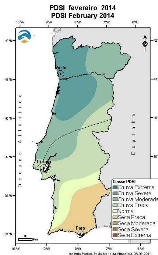
Figura 6 – Distribuição espacial do índice de seca meteorológica em 28 de fevereiro de 2014
