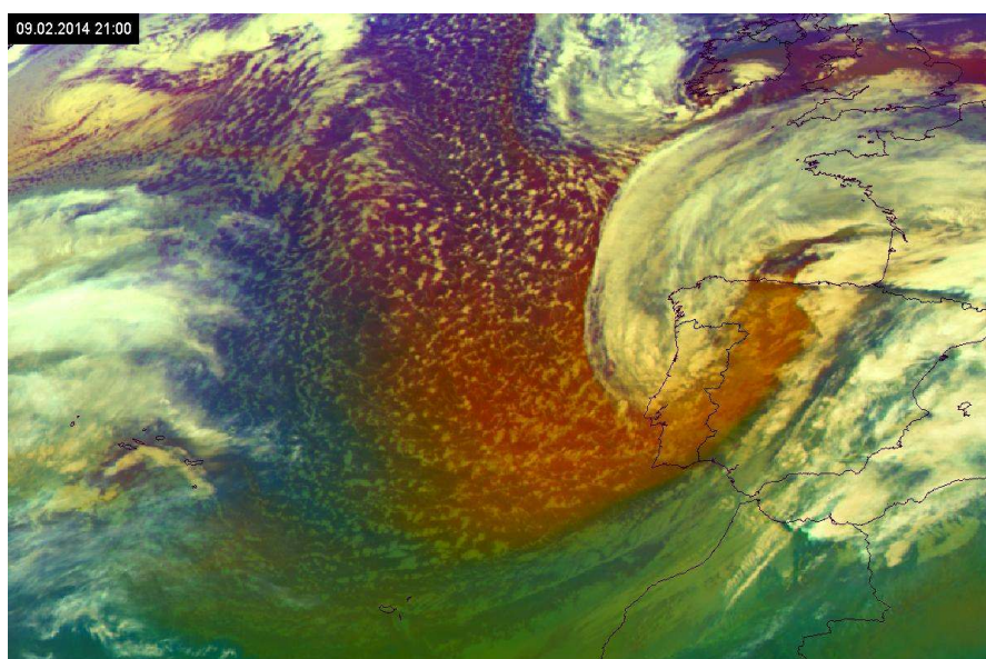
Figura 1 - Imagem RGB Massa de Ar do satélite MSG ( meteosat 2ª geração ) do dia 09 fevereiro 2014 às 21UTC – Tempestade Stephanie
