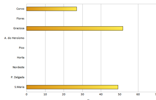
Figura 7. Percentagem da irradiação global mensal relativamente ao topo da atmosfera para o mês de setembro de 2021 para várias estações dos Açores.
