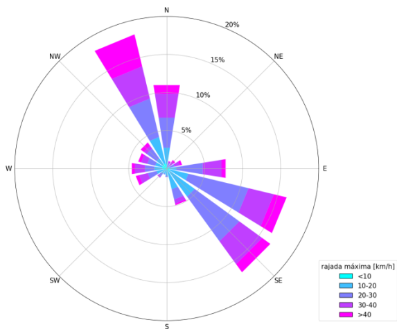
Distribuição de frequências de direção e intensidades de rajada máxima [km/h]. Estação: Sines / Monte Chãos (IPMA); Mês: Dezembro; Ano: 2021
