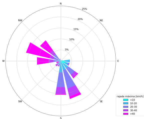
Distribuição de frequências de direção e intensidades de rajada máxima [km/h]. Estação: Lisboa / Geofísico (IPMA); Mês: Dezembro; Ano: 2021
