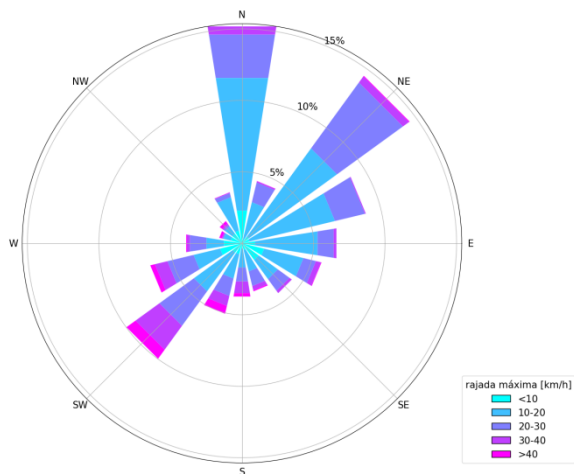
Distribuição de frequências de direção e intensidades de rajada máxima [km/h]. Estação: Beja (IPMA); Mês: Dezembro; Ano: 2021
