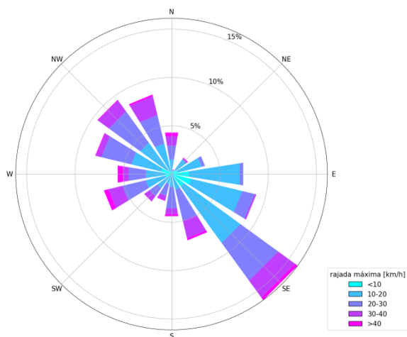
Figura 11. Rosa-dos-Ventos para o mês de dezembro de 2021 nas estação meteorológicas de Bragança, Porto, Guarda, Portalegre, Lisboa, Sines, Beja e Faro
