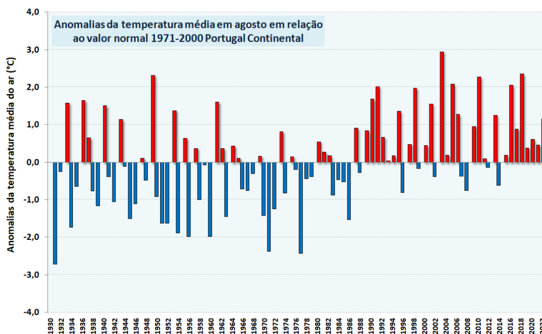
Figura 1. Anomalias da temperatura média do ar no mês de agosto, em Portugal continental, em relação aos valores médios no período 1971-2000
