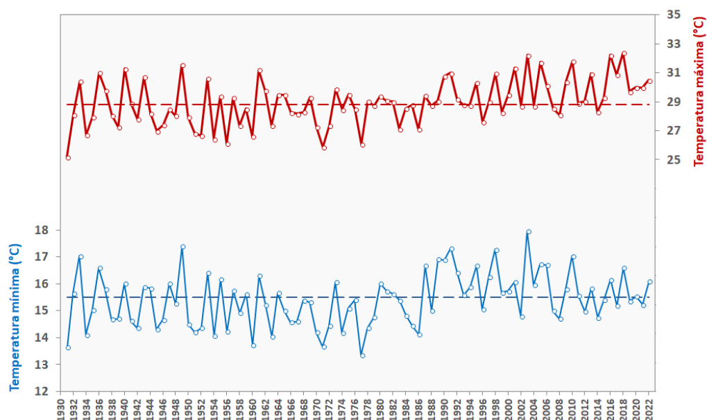
Figura 2. Variabilidade da temperatura máxima e mínima do ar no mês de agosto, em Portugal continental. (Linhas a tracejado indicam a média no período 1971-2000)
