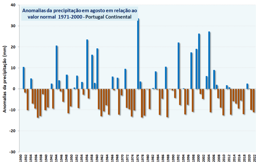
Figura 9. Anomalias da quantidade de precipitação, no mês de agosto, em Portugal continental, em relação aos valores médios no período 1971-2000
