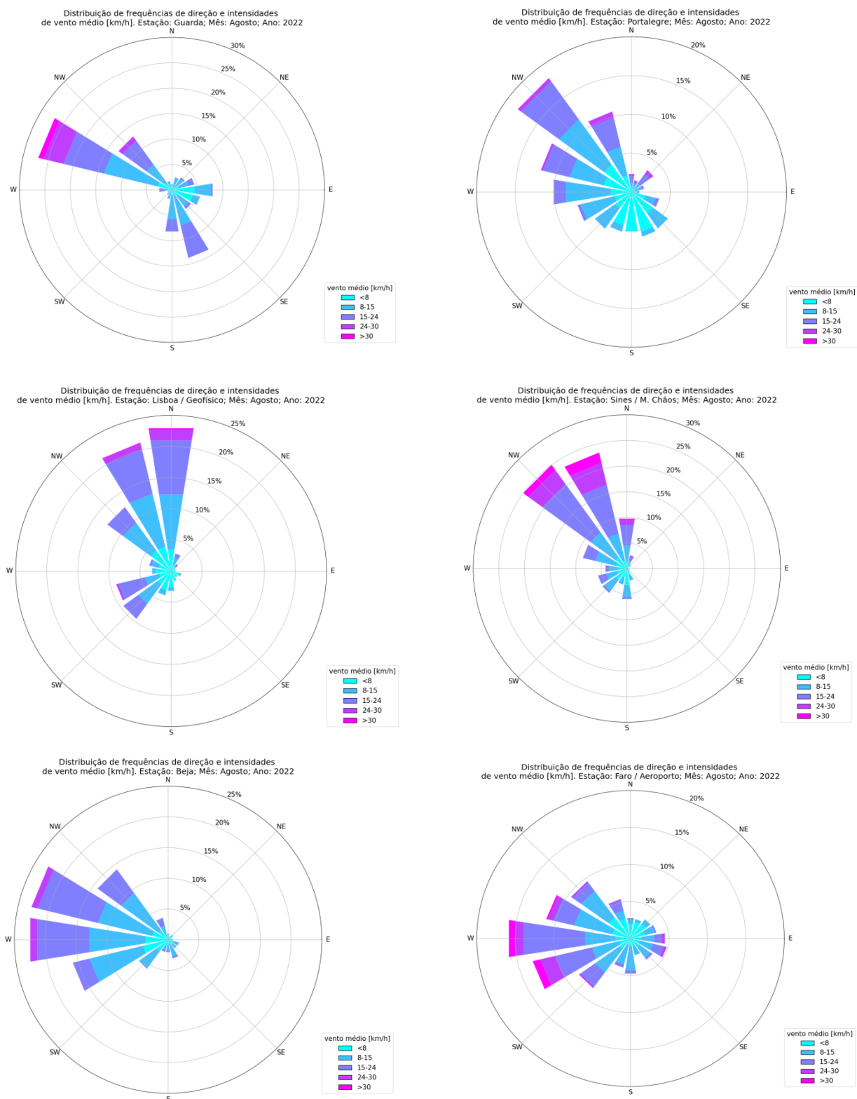
Figura 15. Rosa-dos-Ventos (vento médio) para o mês de agosto de 2022 nas estações meteorológicas de Bragança, Porto, Guarda, Portalegre, Lisboa, Sines, Beja e Faro
