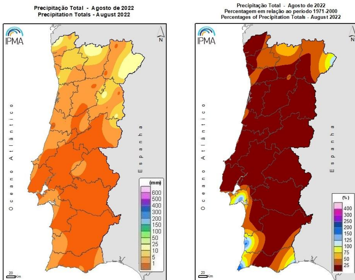
Figura 10. Distribuição espacial da precipitação total e respetiva percentagem em relação à média (período 1971-2000), no mês de agosto de 2022
