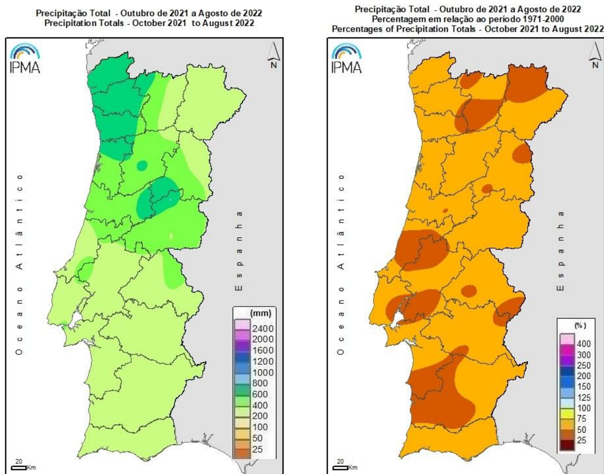
Figura 11. Precipitação acumulada desde 1 de outubro 2021 (esq.) e percentagem em relação à média (dir.)
