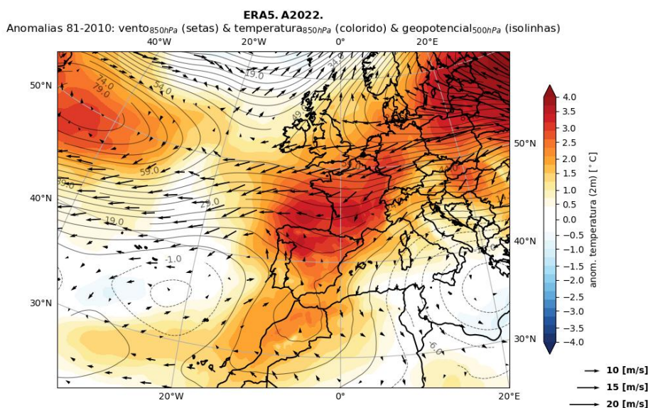
Figura 4. Carta relativa às anomalias (81-10), sobre a região Euro-Atlântica, dos seguintes campos: vento médio (850hPa), temperatura média do ar (850hPa) e geopotencial médio (500hPa) no mês de Agosto de 2022 1
