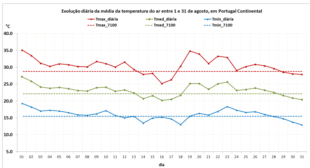
Figura 6. Evolução diária da temperatura do ar de 1 a 31 de agosto de 2022 em Portugal continental
