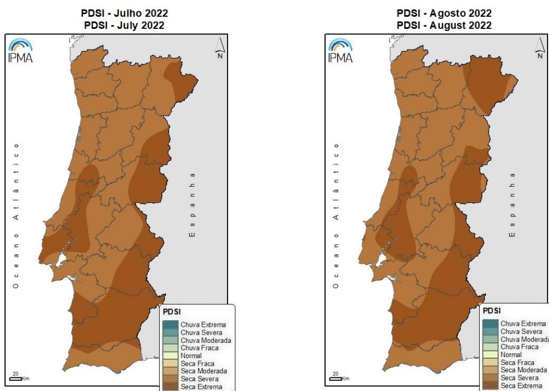
Figura 13. Distribuição espacial do índice de seca meteorológica a 31 julho e a 31 agosto
