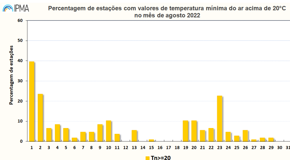
Figura 8. Percentagem de estações com valores de temperatura mínima do ar \geq 20^{\circ}\text{C} observados em agosto 2022 em Portugal continental (total de estações: 104)
