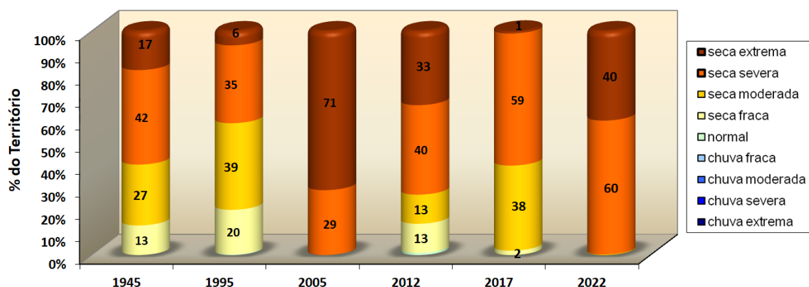
Figura 14. Percentagem do território de Portugal Continental por classe do índice PDSI em situações de seca anteriores em agosto
