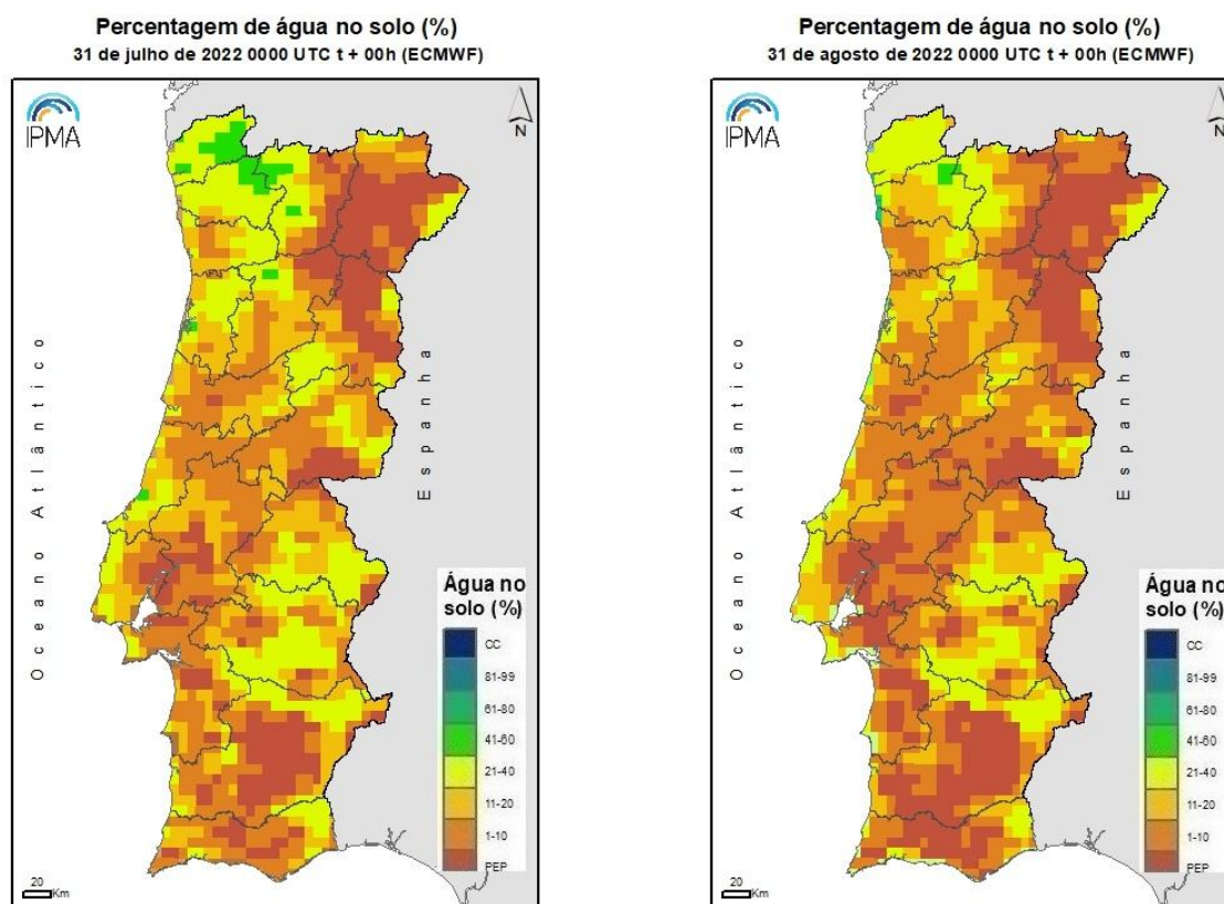
Figura 12. Percentagem de água no solo (média 0-100 cm profundidade), em relação à capacidade de água utilizável pelas plantas (ECMWF) a 31 julho e a 31 de agosto
