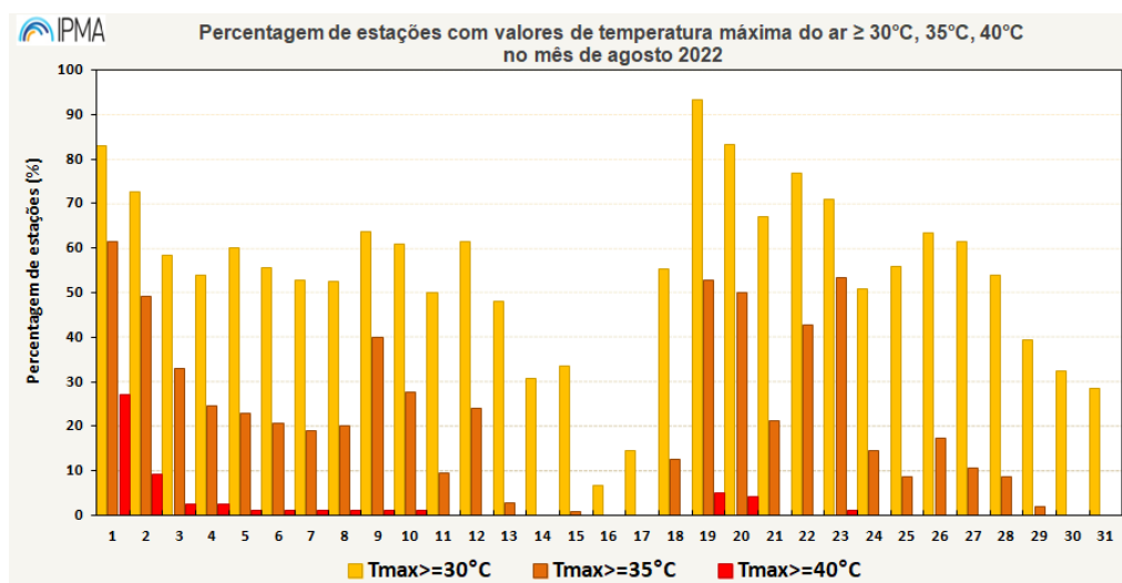
Figura 7. Percentagem de estações com valores de temperatura máxima do ar \geq 30^{\circ}\text{C} , 35^{\circ}\text{C} e 40^{\circ}\text{C} observados em agosto 2022 em Portugal continental (total de estações: 104)
