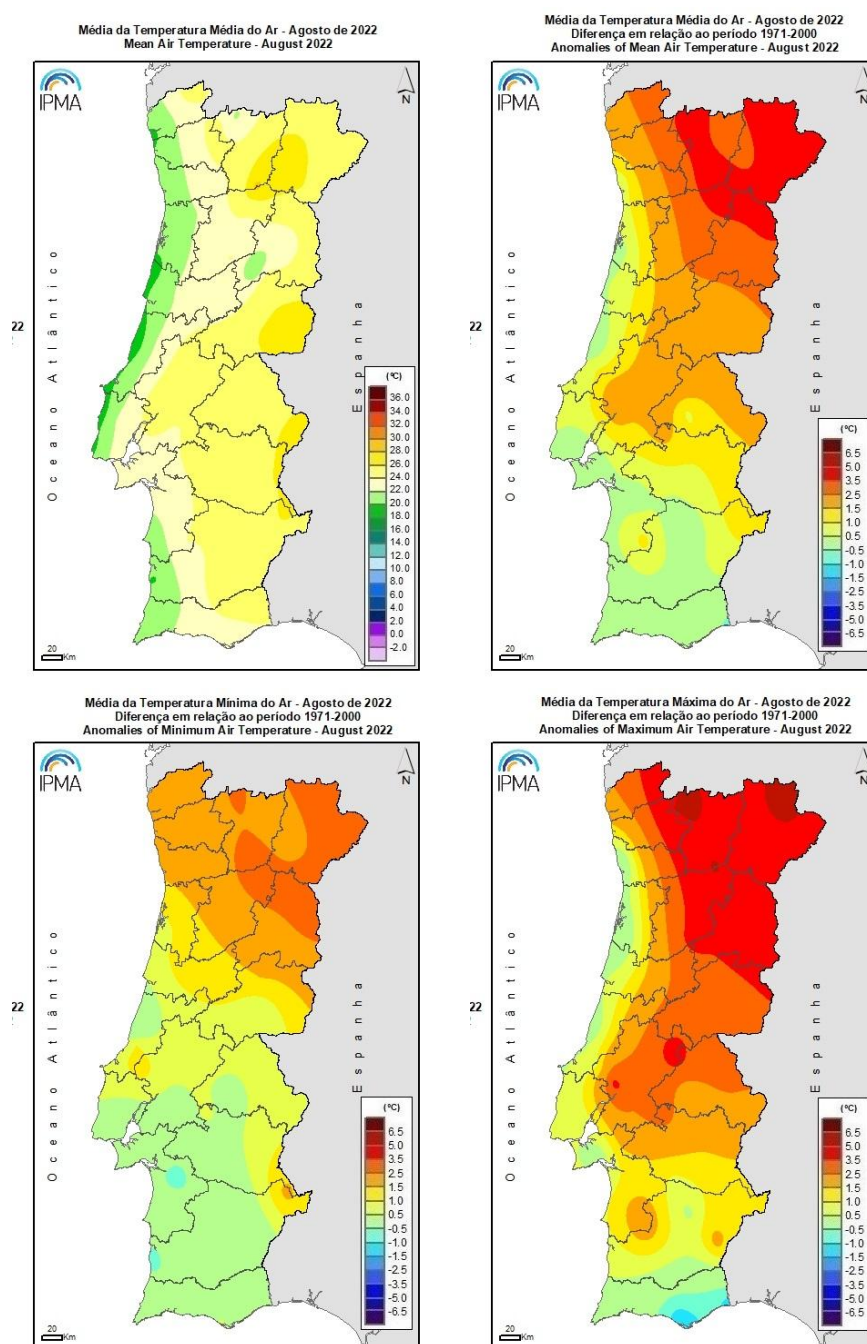
Figura 5. Distribuição espacial dos valores médios da temperatura média do ar e anomalias da temperatura média, mínima e máxima do ar (em relação ao período 1971-2000), no mês de agosto de 2022
