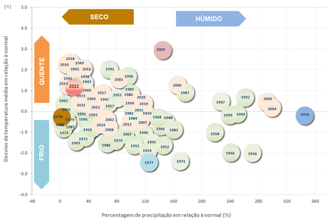
Figura 1. Temperatura do ar e precipitação no mês de agosto (período 1941 – 2022)
