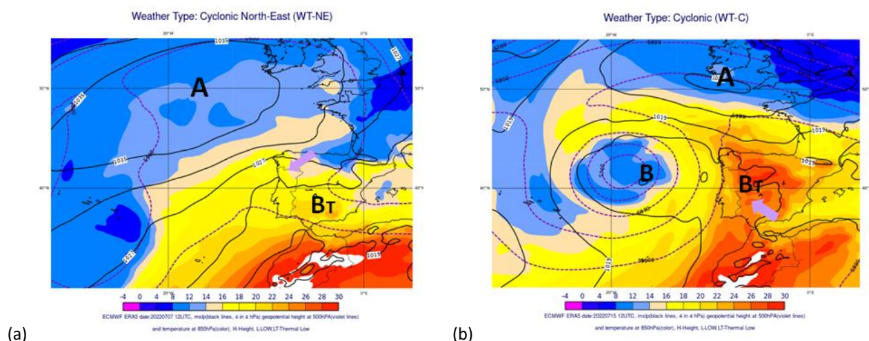
Figura 1 - Tipos de Tempo julho de 2022: ECMWF (ERA5), pressão ao nível médio do mar (linhas a preto, hPa), altura do geopotencial aos 500 hPa (linhas violeta a tracejado, 50 em 50 m), temperatura aos 850 hPa (cor). (a) WT- NE (7 julho), (b) WT - C (15 julho). A- Anticiclone, B- Depressão, B T - Depressão Térmica, seta a violeta - direção do fluxo
