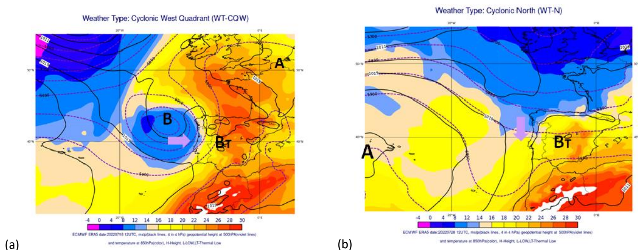
Figura 2 - Tipos de Tempo julho de 2022: ECMWF (ERA5), pressão ao nível médio do mar (linhas a preto, hPa), altura do geopotencial aos 500 hPa (linhas violeta a tracejado, 50 em 50 m), temperatura aos 850 hPa (cor). (a) WT-CQW (18 julho), (b) WT- N (28 julho). A- Anticiclone, B- Depressão, B T - Depressão Térmica, seta a violeta - direção do fluxo
