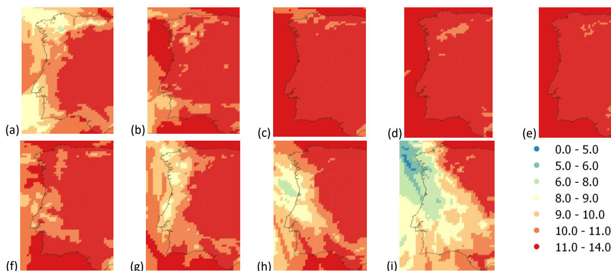
Figura 10 – Anomalia (com base no modelo do ECMWF no período de 2000-2019) do valor máximo do índice de Haines Contínuo em julho de 2022, (a) dia 10, (b) dia 11, (c) dia 12, (d) dia 13, (e) dia 14, (f) dia 15, (g) dia 16, (h) dia 17, (i) dia 18.
