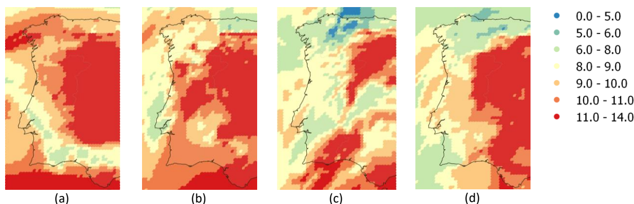
Figura 10 – Anomalia (com base no modelo do ECMWF no período de 2000-2019) do valor máximo do índice de Haines Contínuo em agosto de 2022, (a) dia 1, (b) dia 3, (c) dia 13, (d) dia 23,
