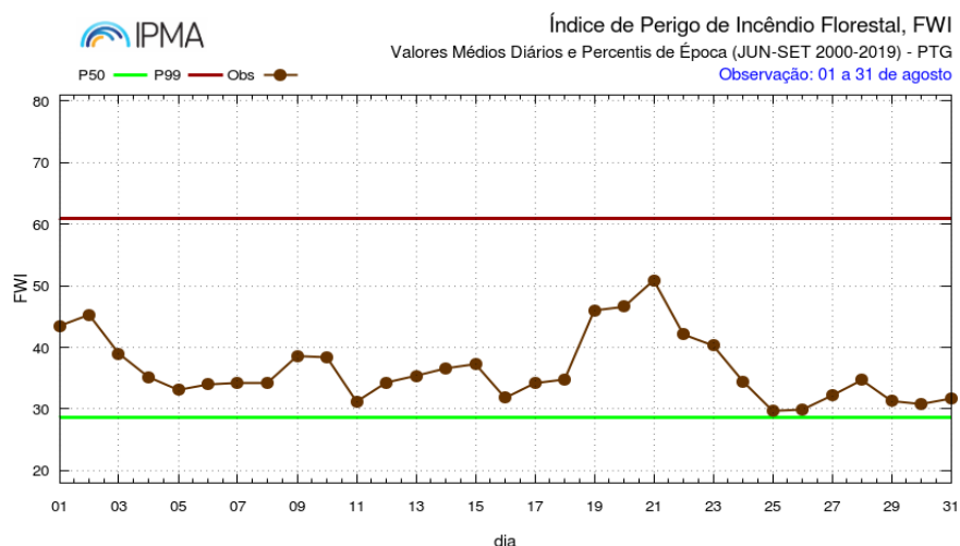
Figura 7 - Evolução diária dos índices dos combustíveis finos (FFMC), propagação inicial (ISI) e do índice meteorológico de perigo de incêndio, FWI e comparação com os percentis do período de 1 junho a 30 setembro. (a) Valor médio diário em Portugal continental (CONT), (a) FFMC, (b) ISI, (c) FWI.
