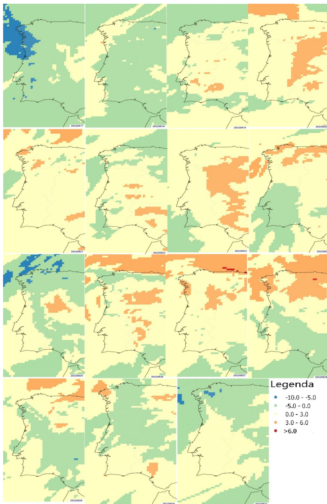
Figura AIV.2 – Mapas das anomalias do valor máximo diário do Índice Contínuo de Haines , agosto de 2022 (16 a 31).
