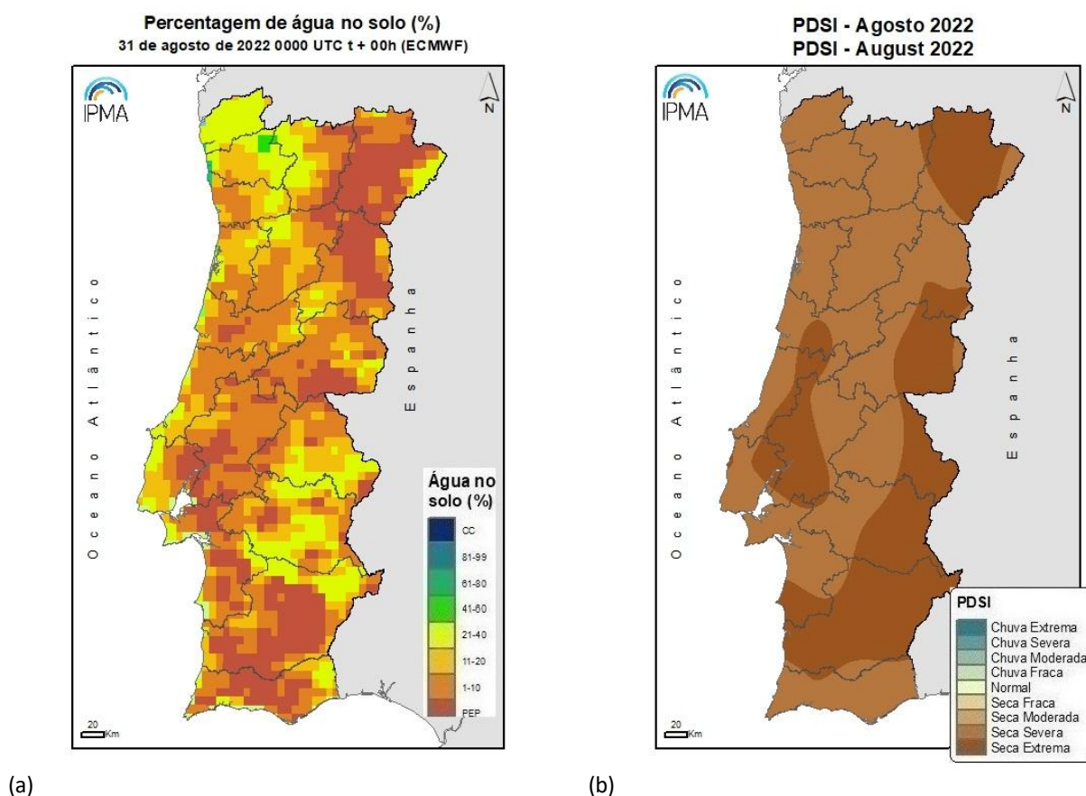
Figura 4 - Distribuição espacial em 31 de agosto de 2022 do teor de Água no Solo e da Seca, (a) percentagem de água no solo (média 0-100 cm profundidade), em relação à capacidade de água utilizável pelas plantas (ECMWF), (b) índice de seca, PDSI.
