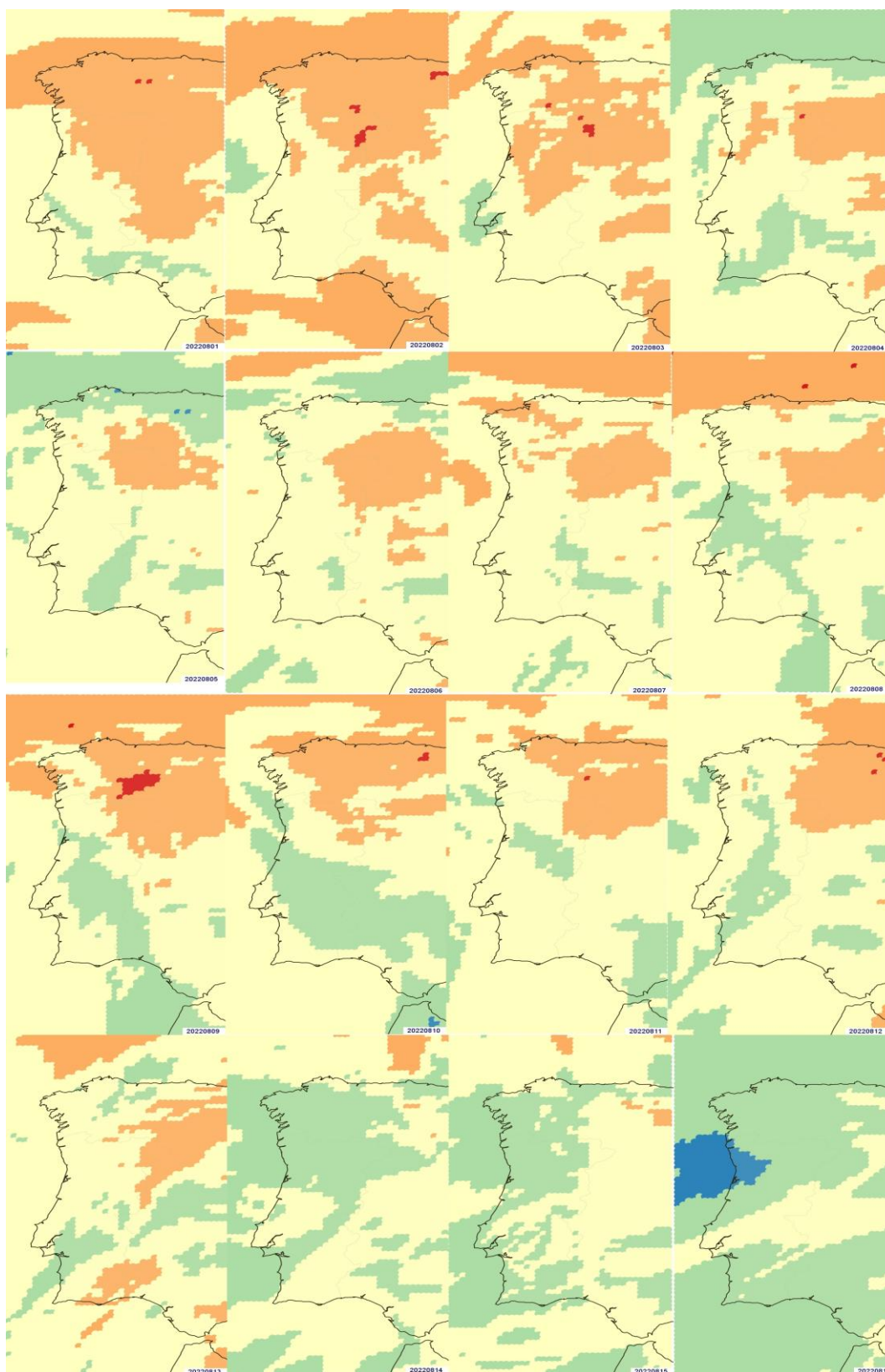
Figura AIV.1 – Mapas das anomalias do valor máximo diário do Índice Contínuo de Haines , agosto de 2022 (1 a 16).
