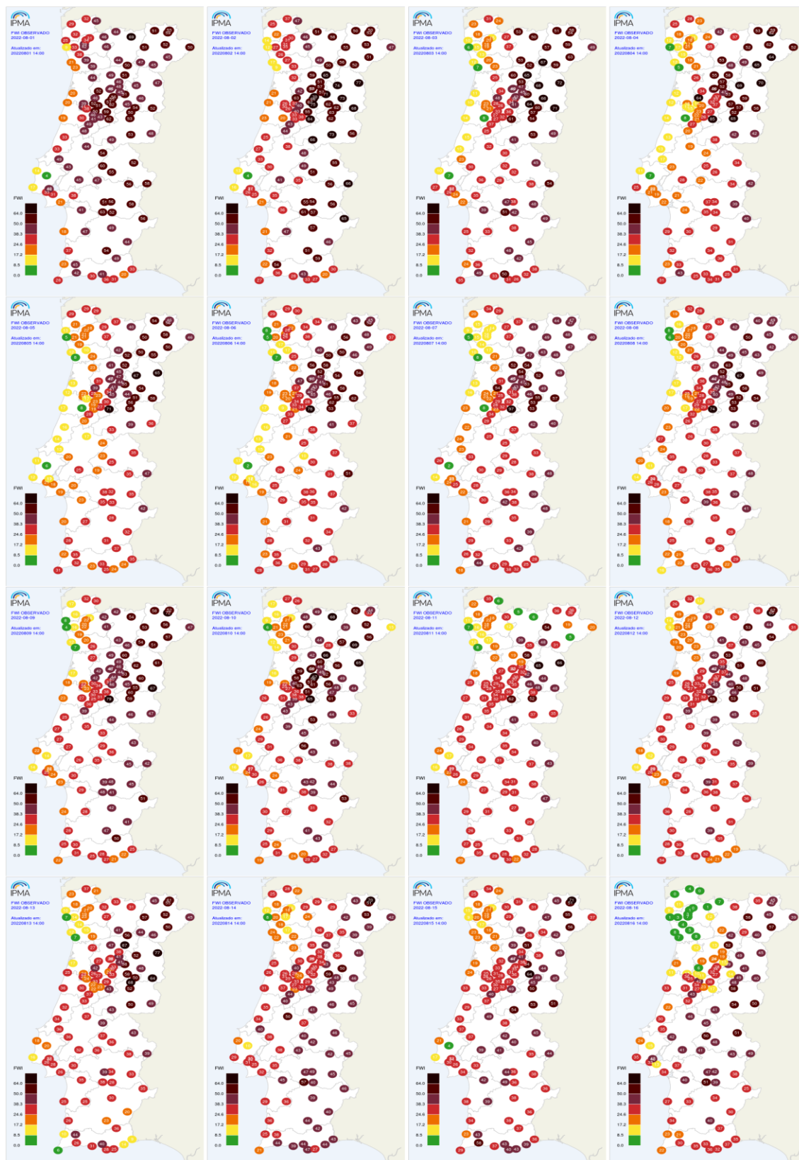
Figura AII.1 – Mapas do FWI Observado nas estações meteorológicas, agosto de 2022 (dias 1 a 16).
