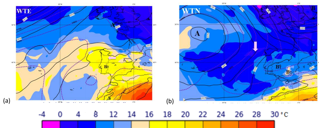
Figura 2 - Tipos de Tempo setembro de 2022: ECMWF (ERA5), pressão ao nível médio do mar 12 UTC (linhas a preto, 4 em 4 hPa), altura do geopotencial aos 500 hPa (linhas violeta a tracejado, 50 em 50 m), temperatura aos 850 hPa (cor). (a) WT-E (20 setembro), (b) WTN (26 setembro). A- Anticiclone, B- Depressão, B T . Depressão Térmica, seta rosa - direção do fluxo.
