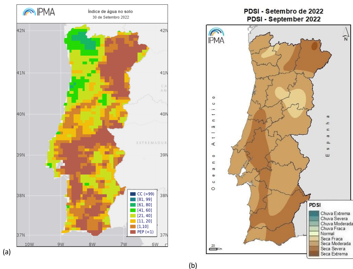
Figura 4 - Distribuição espacial em 30 de setembro de 2022 do teor de Água no Solo e da Seca, (a) percentagem de água no solo (média 0-100 cm profundidade), em relação à capacidade de água utilizável pelas plantas (ECMWF), (b) índice de seca, PDSI.
