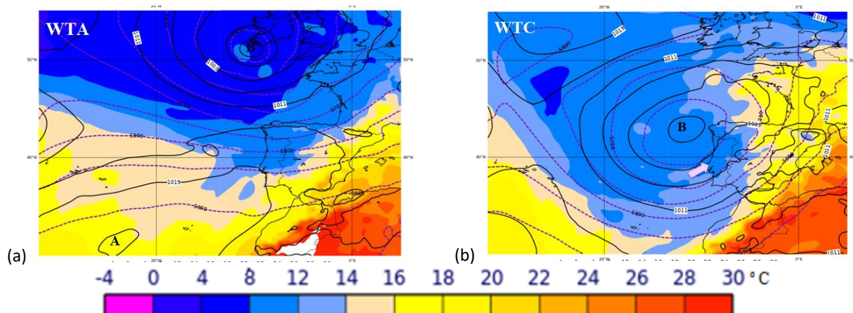
Figura 1 - Tipos de Tempo setembro de 2022: ECMWF (ERA5), pressão ao nível médio do mar 12 UTC (linhas a preto, 4 em 4 hPa), altura do geopotencial aos 500 hPa (linhas violeta a tracejado, 50 em 50 m), temperatura aos 850 hPa (cor). (a) WT-A (7 setembro), (b) WT-C (13 setembro). A- Anticiclone, B- Depressão, B T . Depressão Térmica, seta rosa - direção do fluxo
