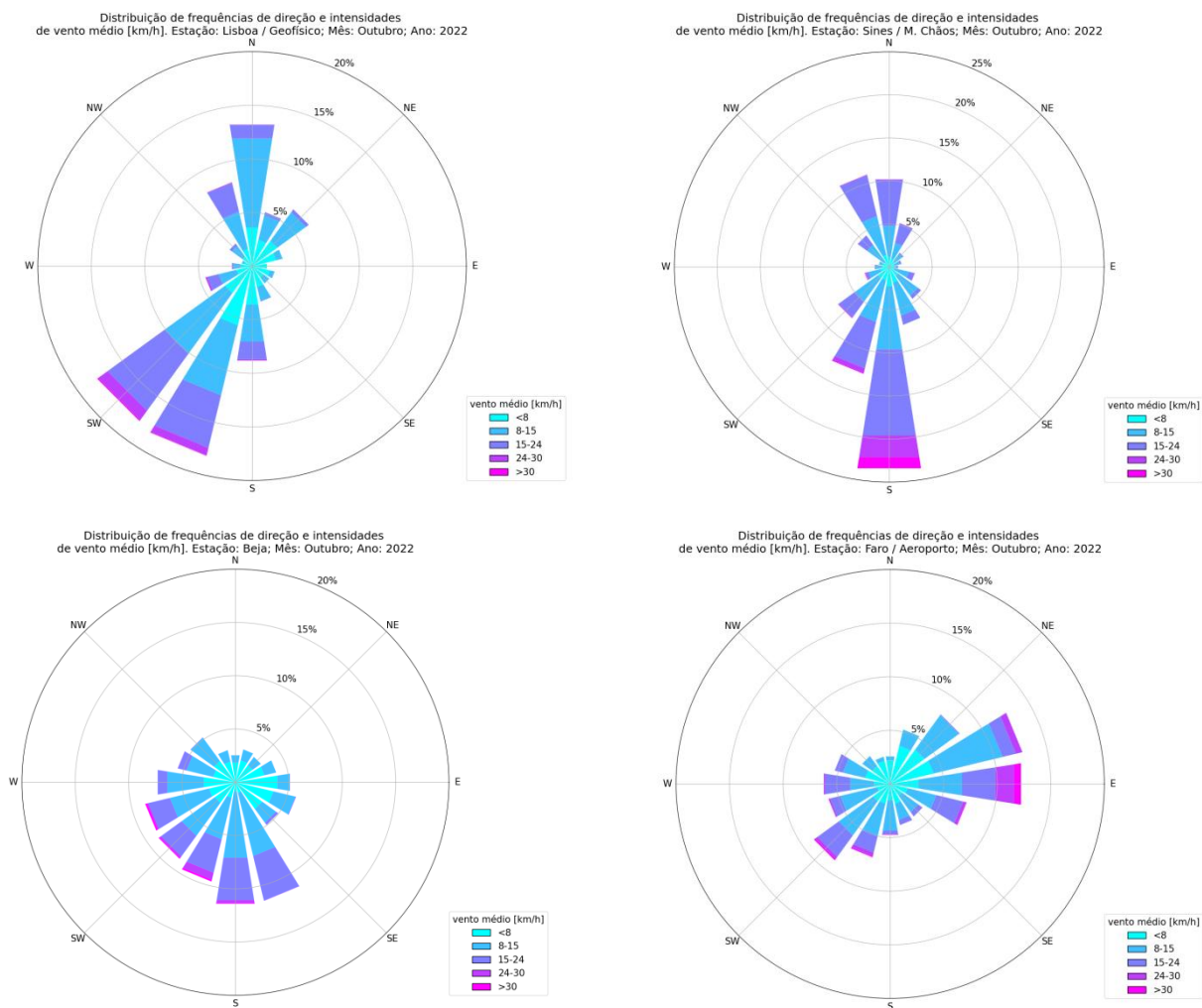
Figura 12. Rosa-dos-Ventos (vento médio) para o mês de outubro de 2022 nas estações meteorológicas de Bragança, Porto, Guarda, Portalegre, Lisboa, Sines, Beja e Faro
