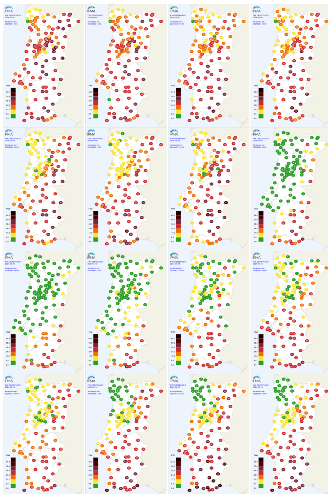
Figura AII.1 – Mapas do FWI Observado nas estações meteorológicas, junho de 2024 (dias 1 a 16).
