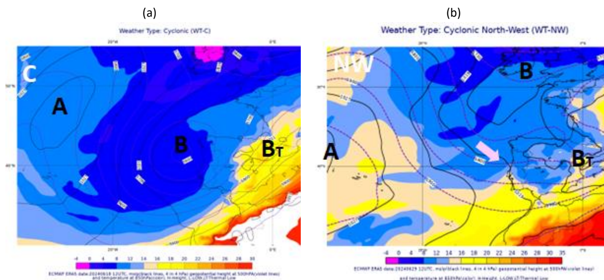
Figura 2 - Tipos de Tempo junho de 2024: ECMWF(ERA5) às 12 UTC. Pressão ao nível médio do mar (linhas a preto, 4 em 4 hPa), altura do geopotencial aos 500 hPa (linhas violeta a tracejado, 50 em 50 m), temperatura aos 850 hPa (cor, °C). (a) WTC (ciclónico, 18 junho), (b) WTNN (fluxo de noroeste, 29 junho). A- Anticiclone, B- Depressão, B T - Depressão Térmica, seta a violeta - direção do fluxo.
