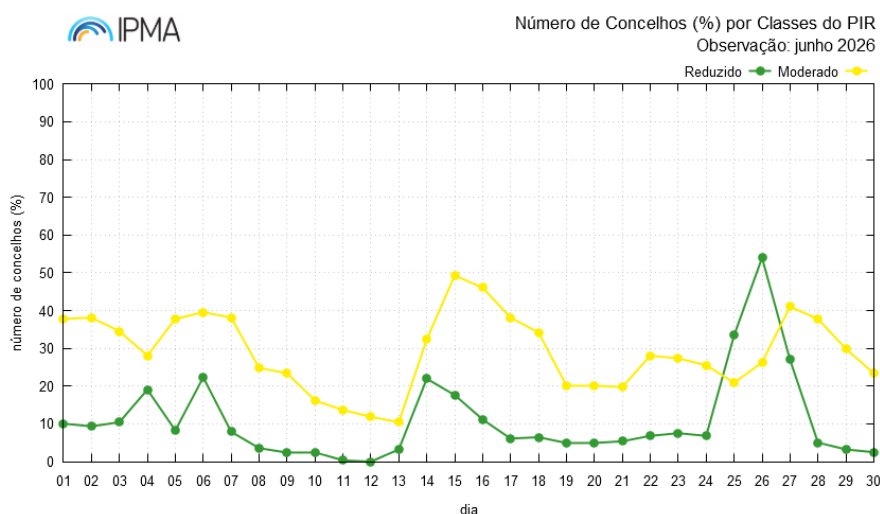
Figura 10- Evolução diária em junho da percentagem de concelhos nas classes de PIR.
