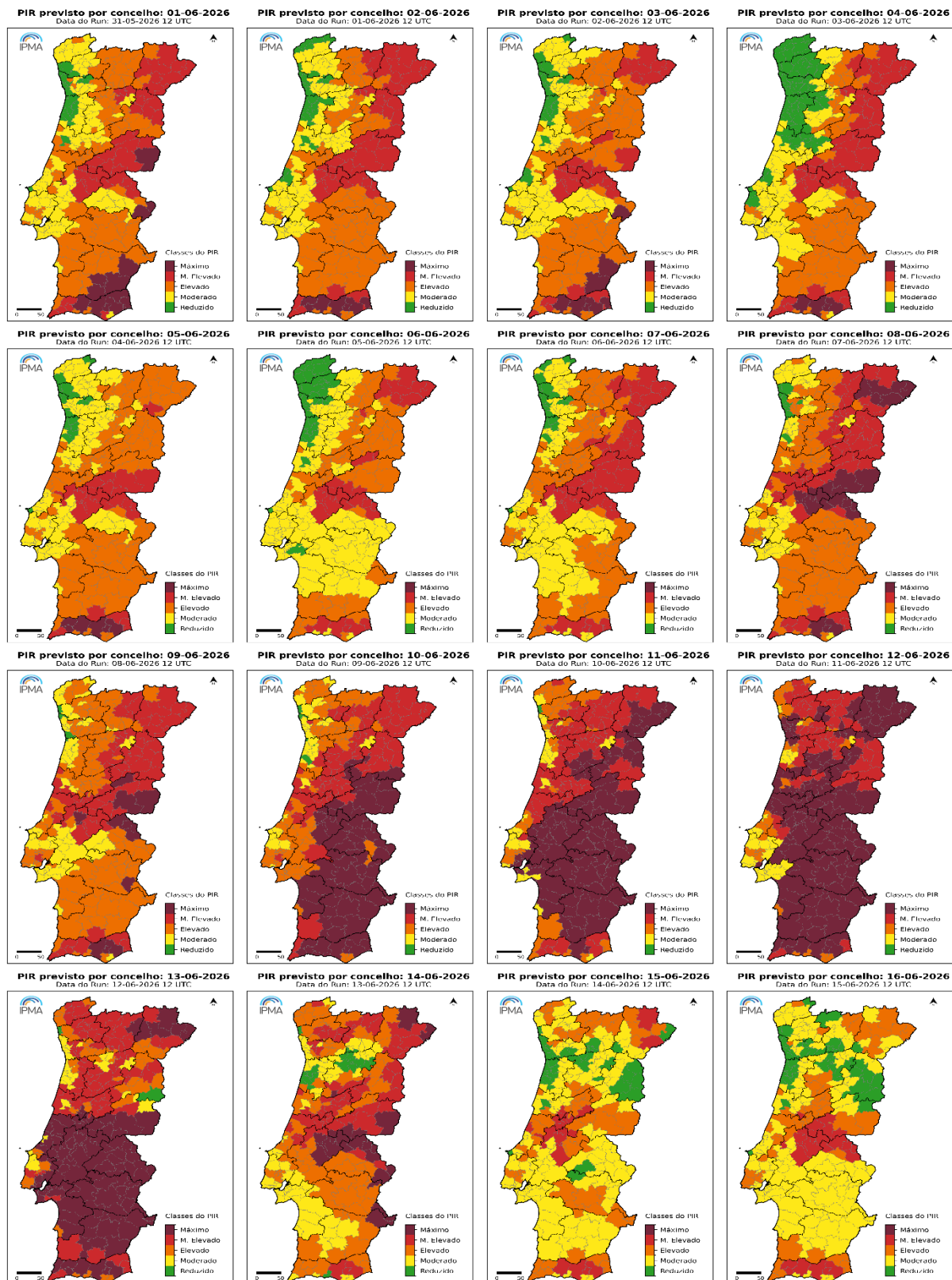
Figura AIV.3 – Mapas das classes de PIR, previsão a nível de Concelho, junho de 2026 (dias 1 a 16).
