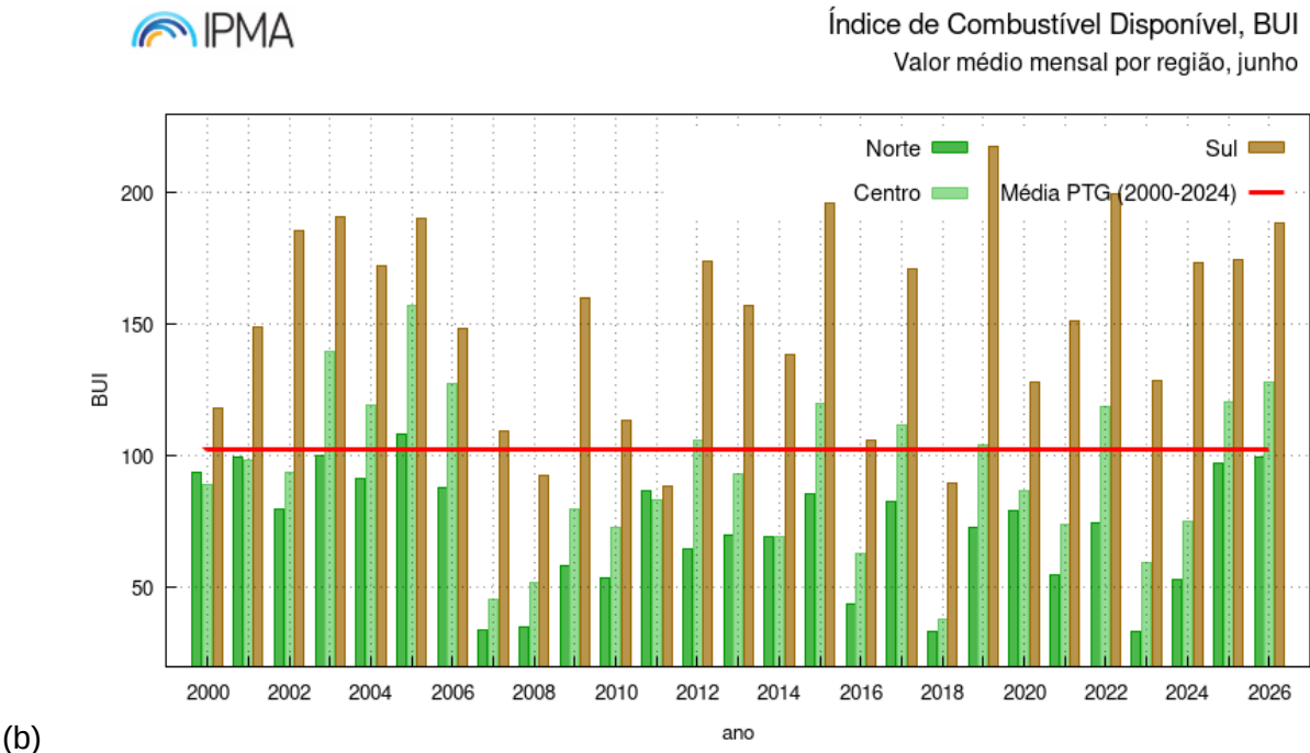
Figura 6 -Valor médio do índice de combustível disponível, BUI. (a)Valor médio do índice de combustível disponível em Portugal continental (CONT), (b) Valor médio do índice de combustível disponível na Região Norte (RN), Região Centro (RC) e Região Sul (RS).
