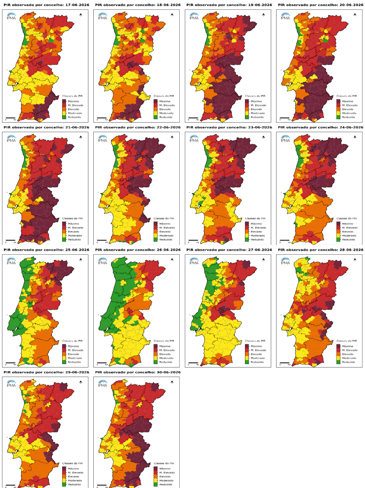
Figura AIV.2 – Mapas das classes de PIR observado a nível de Concelho, junho de 2026 (dias 17 a 30).
