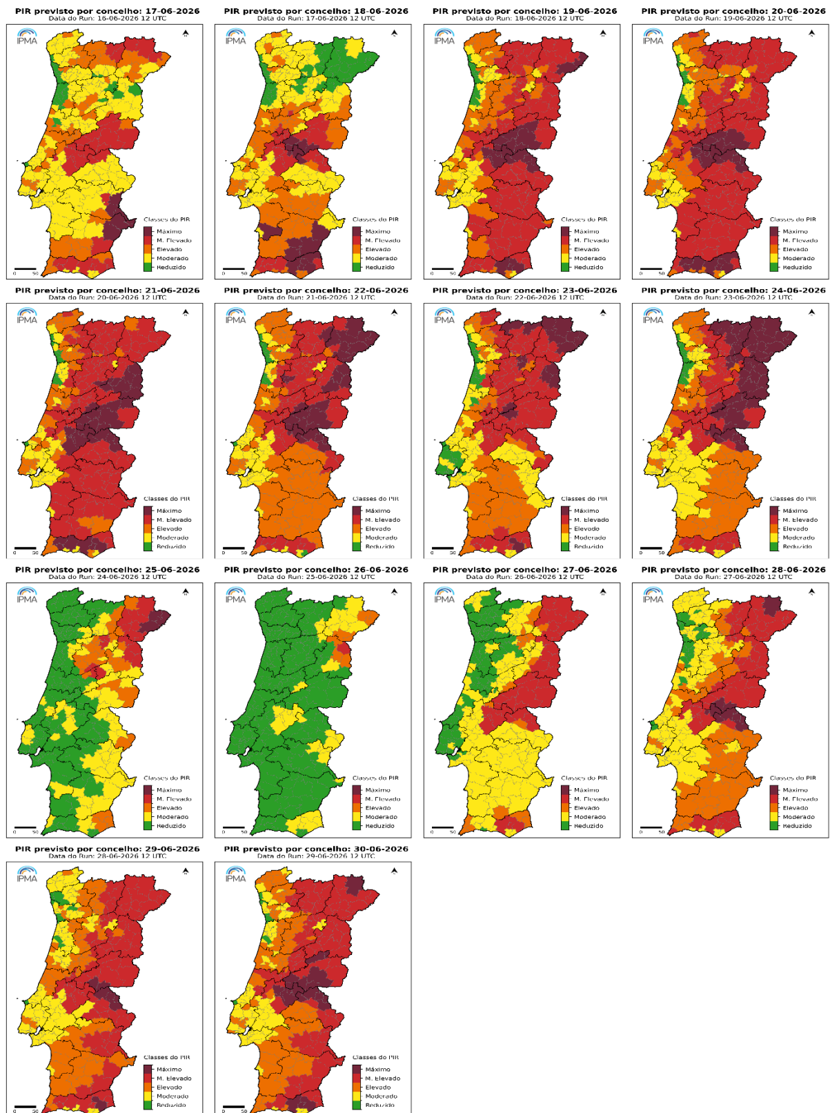
Figura AIV.4 – Mapas das classes de PIR, previsão a nível de Concelho, junho de 2026 (17 a 30).
