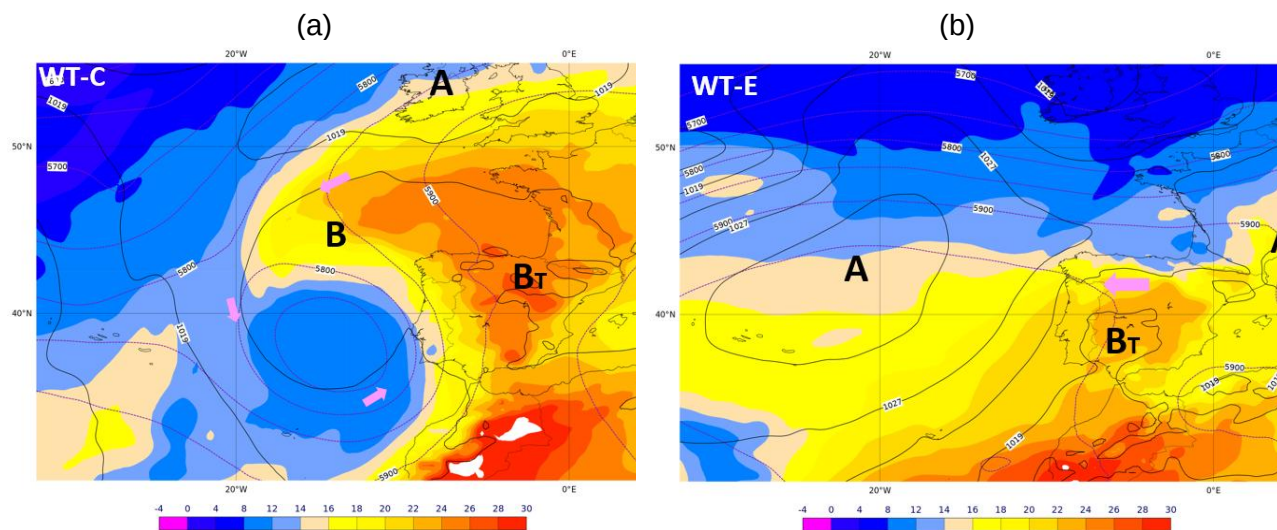
Figura 2- Tipos de Tempo junho de 2026: ECMWF(ERA5) às 12 UTC.
