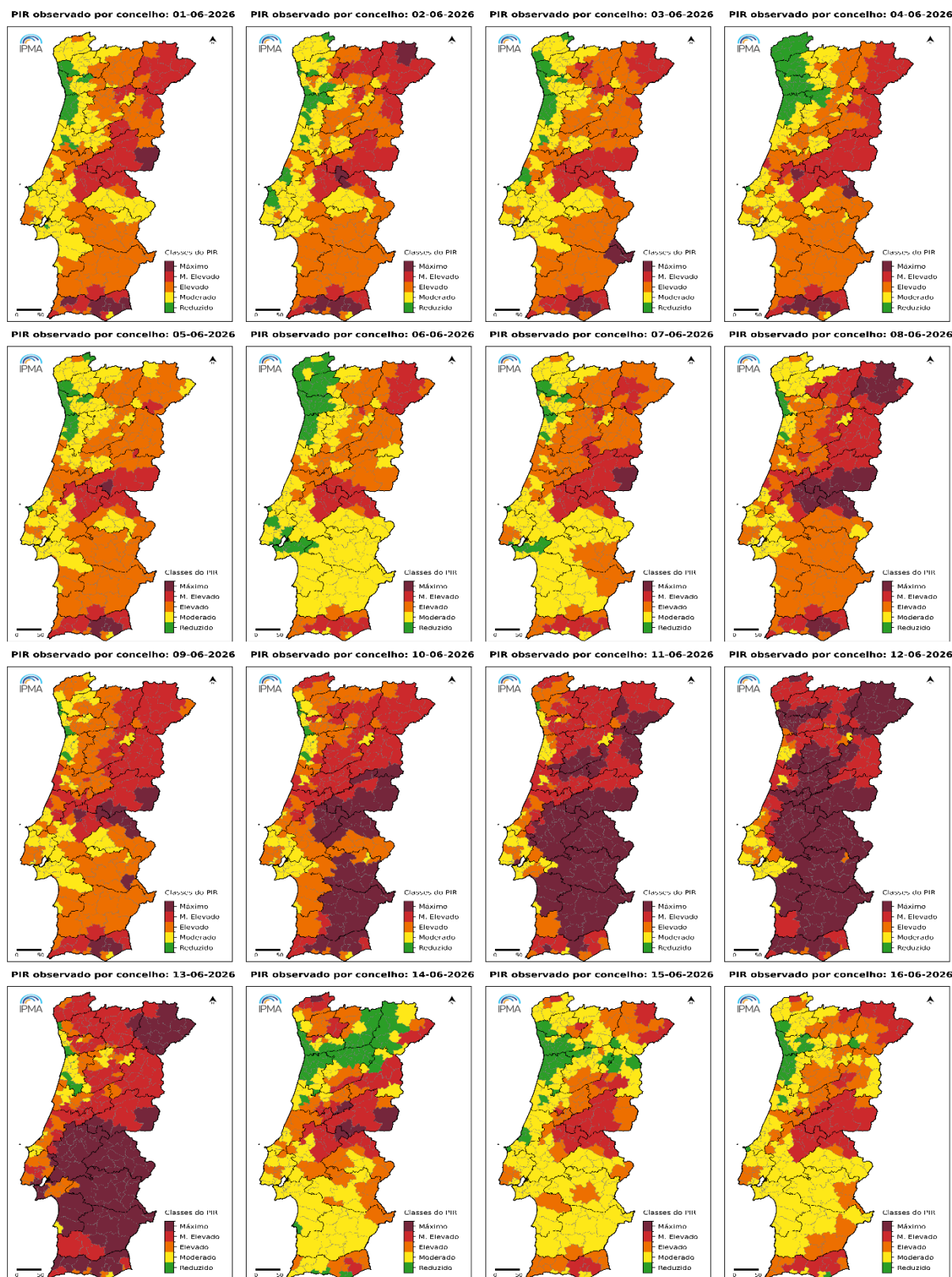
Figura AIV.1 – Mapas das classes de PIR observado a nível de Concelho, junho de 2026 (dias 1 a 16).
