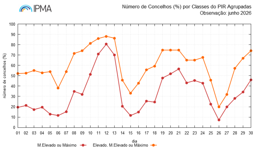
Figura 9- Evolução diária em junho da percentagem de concelhos por classe agrupadas do PIR.
