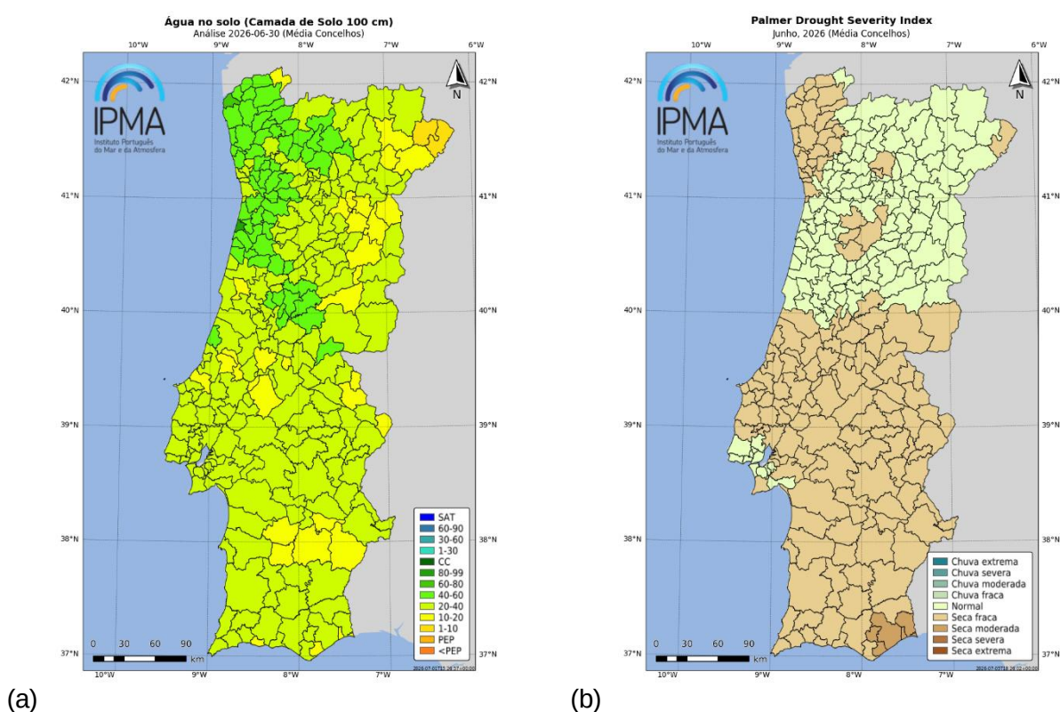
Figura 4- Distribuição espacial em 30 de junho de 2026 do teor de Água no Solo e da Seca (a) percentagem de água no solo (média 0-100 cm profundidade), em relação à capacidade de água utilizável pelas plantas (ECMWF), (b) índice de seca, PDSI.
