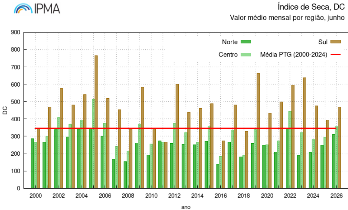
Figura 5 - Valor médio dos índices de seca, DC. (a) Valor médio do índice de seca, DC, em Portugal continental (CONT), (b) Valor médio do índice de seca na Região Norte (RN), Região Centro (RC) e Região Sul (RS).
