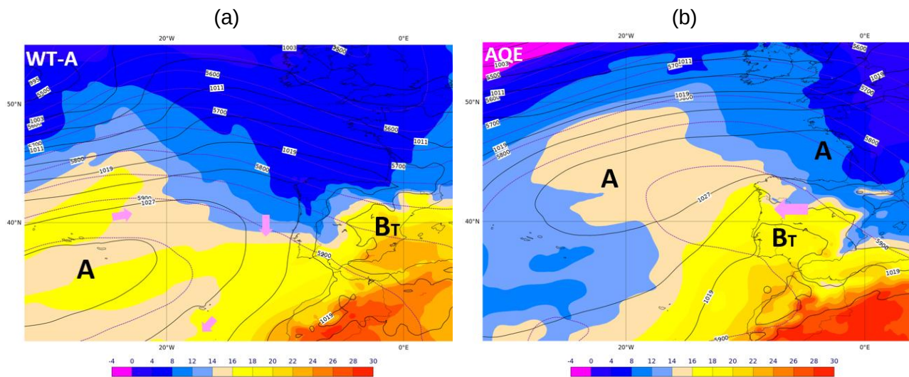
Figura 1- Tipos de Tempo em junho de 2026: ECMWF(ERA5) às 12 UTC.
